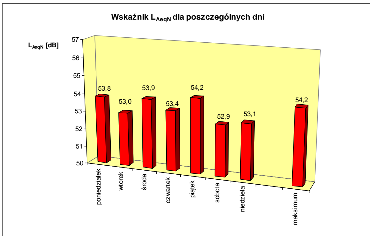
Ryc. 6. Wskaźnik L_{AeqN} (8 h). Zestawienie zmian wskaźnika poziomu hałasu ( L_{AeqN} ), w danym dniu tygodnia oraz jego wartość maksymalna w badanym punkcie, Ślemień 2013 r.
