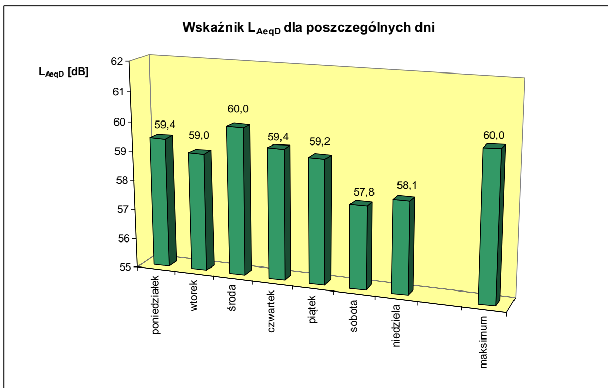
Ryc. 5. Wskaźnik L_{AeqD} (16 h). Zestawienie zmian wskaźnika poziomu hałasu ( L_{AeqD} ), w danym dniu tygodnia oraz jego wartość maksymalna w badanym punkcie, Ślemień 2013 r.
