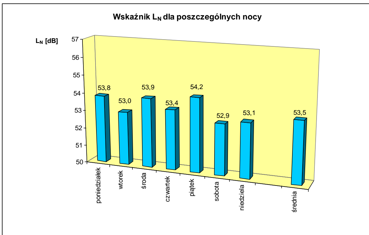
Ryc. 4. Wskaźnik L_N^{1n} (8 h) w [dB]. Zestawienie zmian średniego wskaźnika poziomu hałasu ( L_N ) dla danej nocy tygodnia w badanym punkcie, Ślemień 2013 r.
