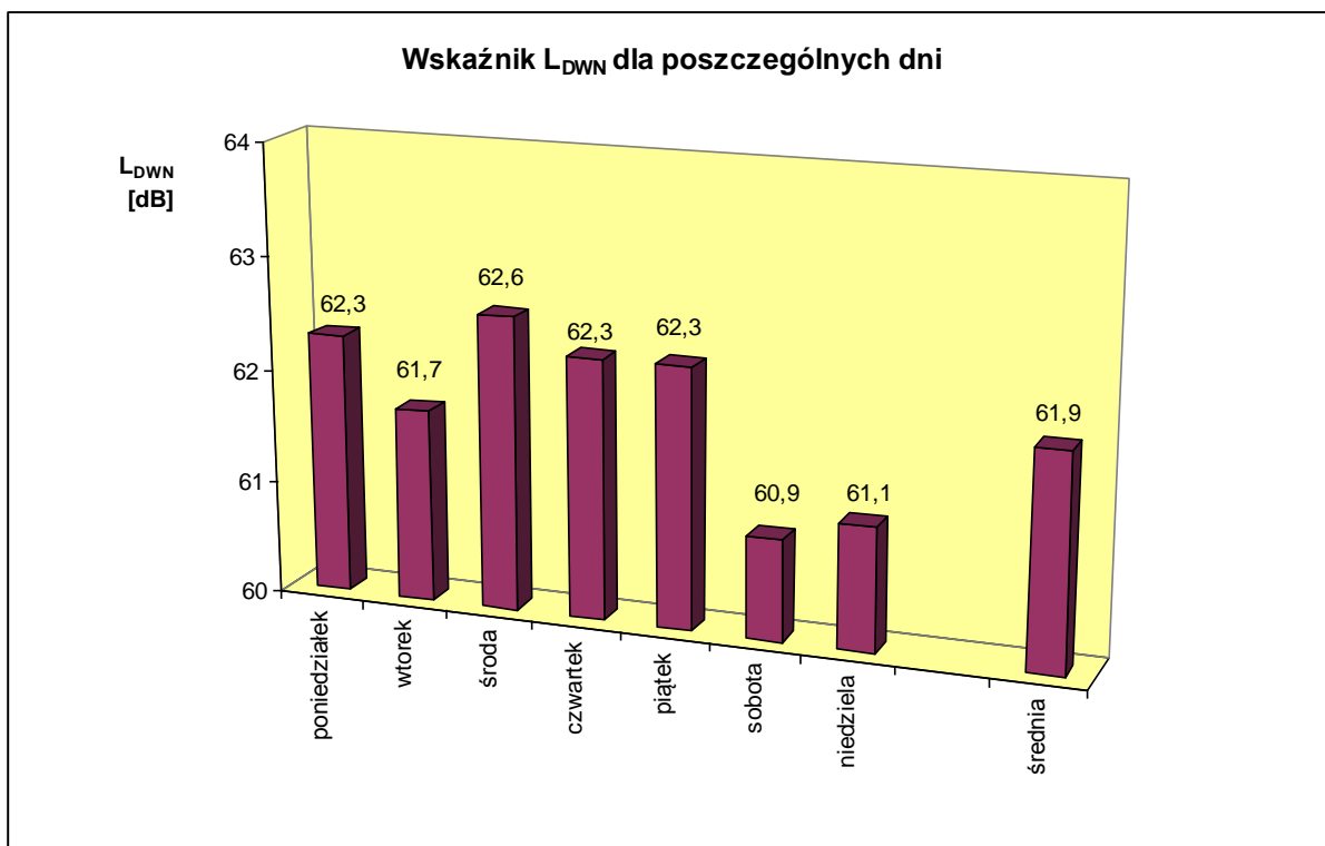
Ryc. 3. Wskaźnik L_{DWN}^{1d} (24 h) w [dB]. Zestawienie zmian średniego wskaźnika poziomu hałasu ( L_{DWN} ) dla danej doby tygodnia w badanym punkcie, Ślemień 2013 r.
