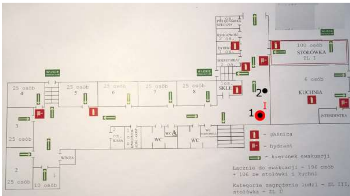
Rys. 1b: Plan rozmięszczenia punktów pomiarowych – parter, kolorem czerwonym oznaczono lokalizację punktów dostępnych
