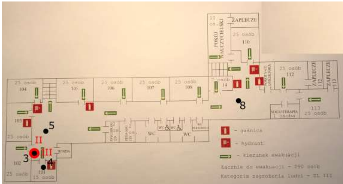
Rys. 1c: Plan rozmieszczenia punktów pomiarowych – I piętro, kolorem czerwonym oznaczono lokalizację punktów dostępowych
