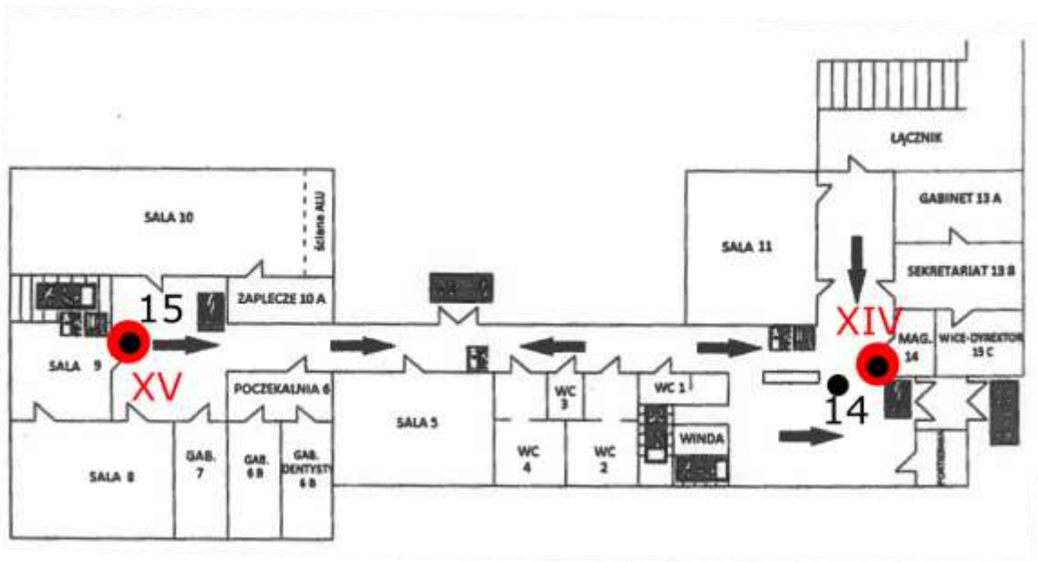
Rys. 1f: Plan rozmieszczenia punktów pomiarowych – 1 piętro, kolorem czerwonym oznaczono lokalizację punktów dostępnych
