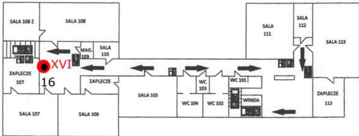
Rys. 1g: Plan rozmieszczenia punktów pomiarowych – 1 piętro, kolorem czerwonym oznaczono lokalizację punktów dostępowych
