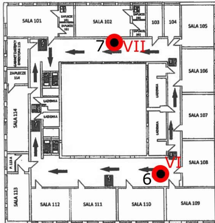
Rys. 1c: Plan rozmieszczenia punktów pomiarowych – 1 piętro, kolorem czerwonym oznaczono lokalizację punktów dostępnych
