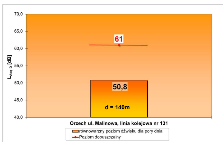
Ryc. 2. Wartość wskaźnika L_{AeqD} dla rozpatrywanego punktu referencyjnego oraz jego porównanie z obowiązującą wartością poziomu dopuszczalnego, Orzech gm. Świerklaniec, 2022 rok.
