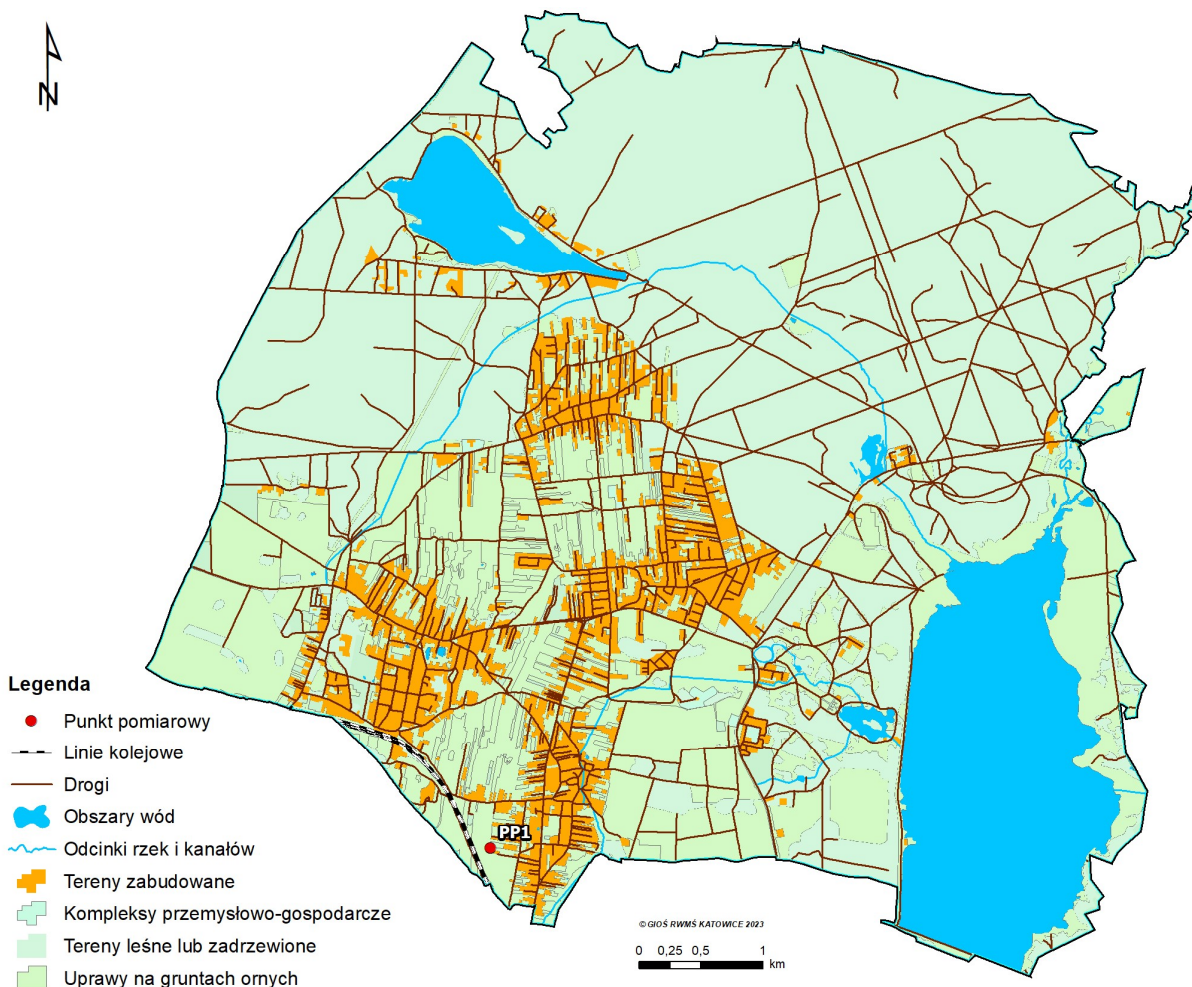
Ryc. 1. Lokalizacja punktu pomiarowego hałasu kolejowego na terenie gminy Świerklaniec.
