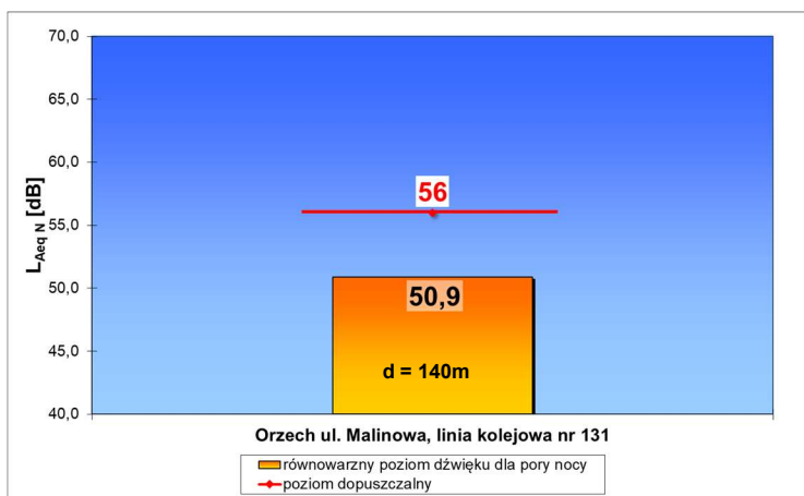
Ryc. 3. Wartość wskaźnika L_{Aeq N} dla rozpatrywanego punktu referencyjnego oraz jego porównanie z obowiązującą wartością poziomu dopuszczalnego, Orzech gm. Świerklaniec, 2022 rok.
