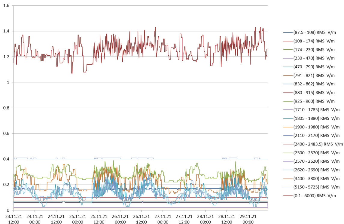
Rys. 5 Wyniki pomiarów dla 20 podzakresów częstotliwości – ZOO
