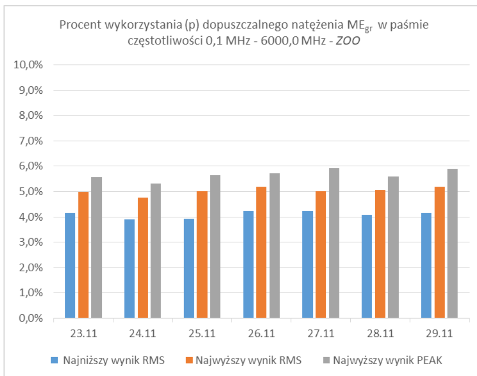
Rys. 26 Procentowe wykorzystanie dopuszczalnego natężenia w zakresie częstotliwości: 0,1 MHz – 6000,0 MHz – ZOO
