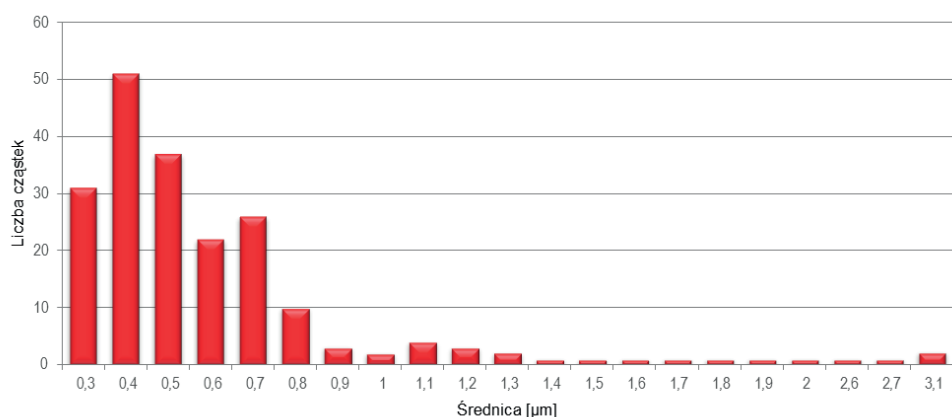
Ryc. 9. Histogram analizy zmian średnicy włókien sącza pustego z włókna szklanego (n = 200)
