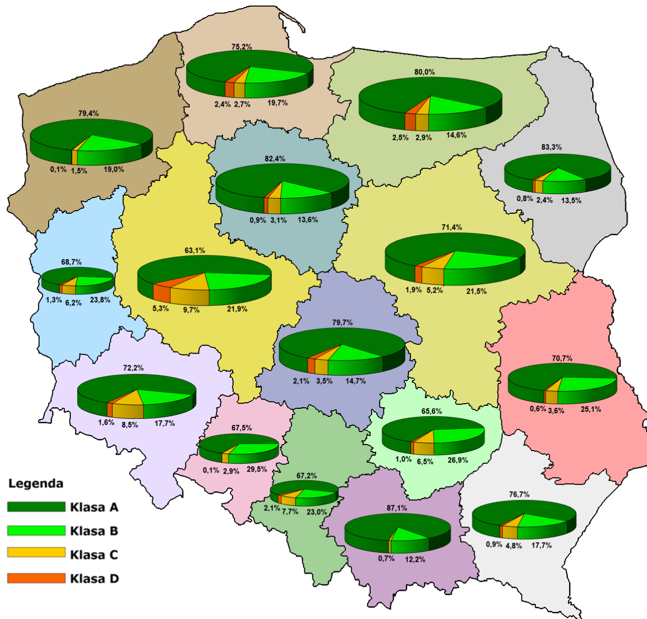
Rysunek 5. Stan techniczny pod względem parametru: koleiny
