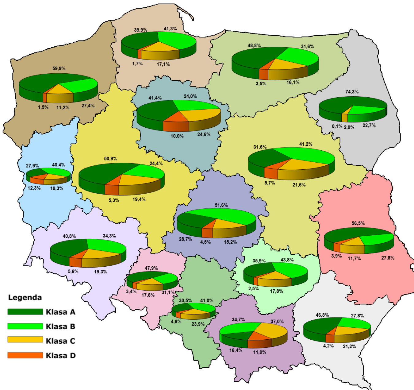
Rysunek 7. Stan techniczny pod względem parametru: współczynnik tarcia
