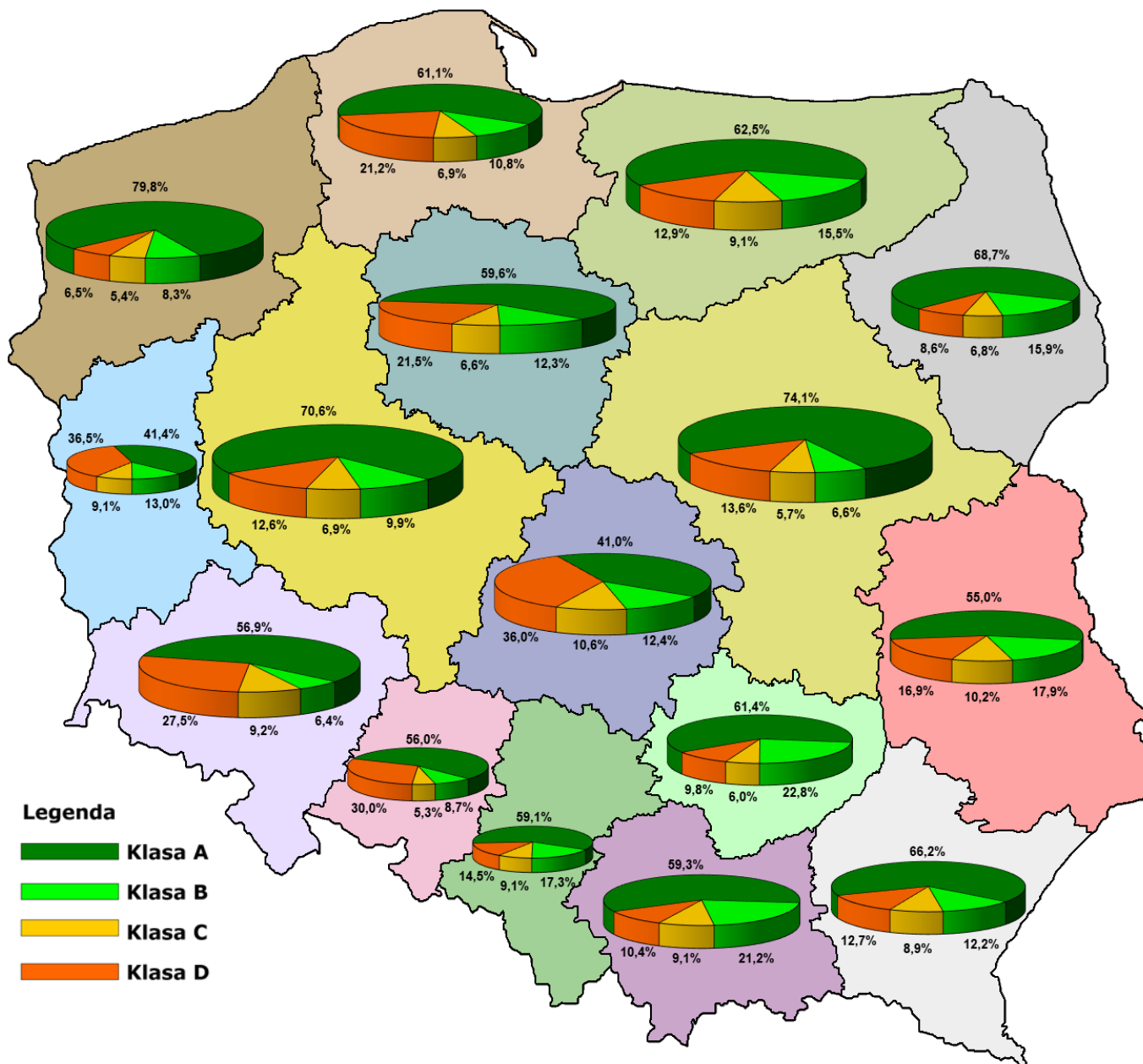
Rysunek 2. Stan techniczny pod względem parametru: wskaźnik ugięć nawierzchni
