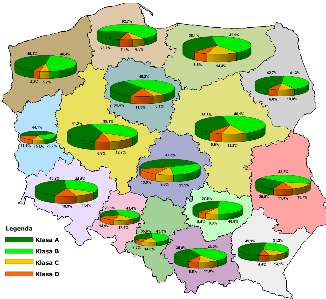
Rysunek 4. Stan techniczny pod względem parametru: pozostała trwałość nawierzchni
