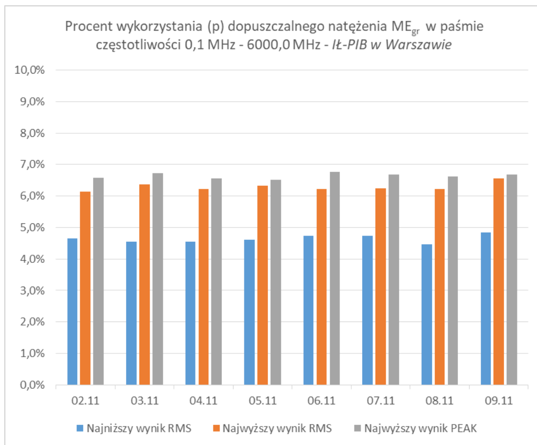
Rys. 25 Procentowe wykorzystanie dopuszczalnego natężenia w zakresie częstotliwości: 0,1 MHz – 6000,0 MHz – It-PIB w Warszawie
