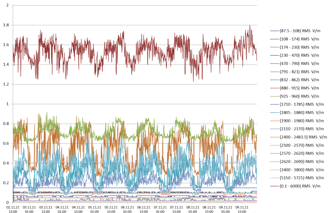
Rys. 4 Wyniki pomiarów dla 20 podzakresów częstotliwości – IŁ-PIB w Warszawie
