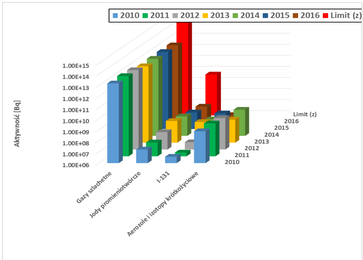
Rysunek 1. Porównanie uwolnień z ostatnich pięciu lat reaktora MARIA.
