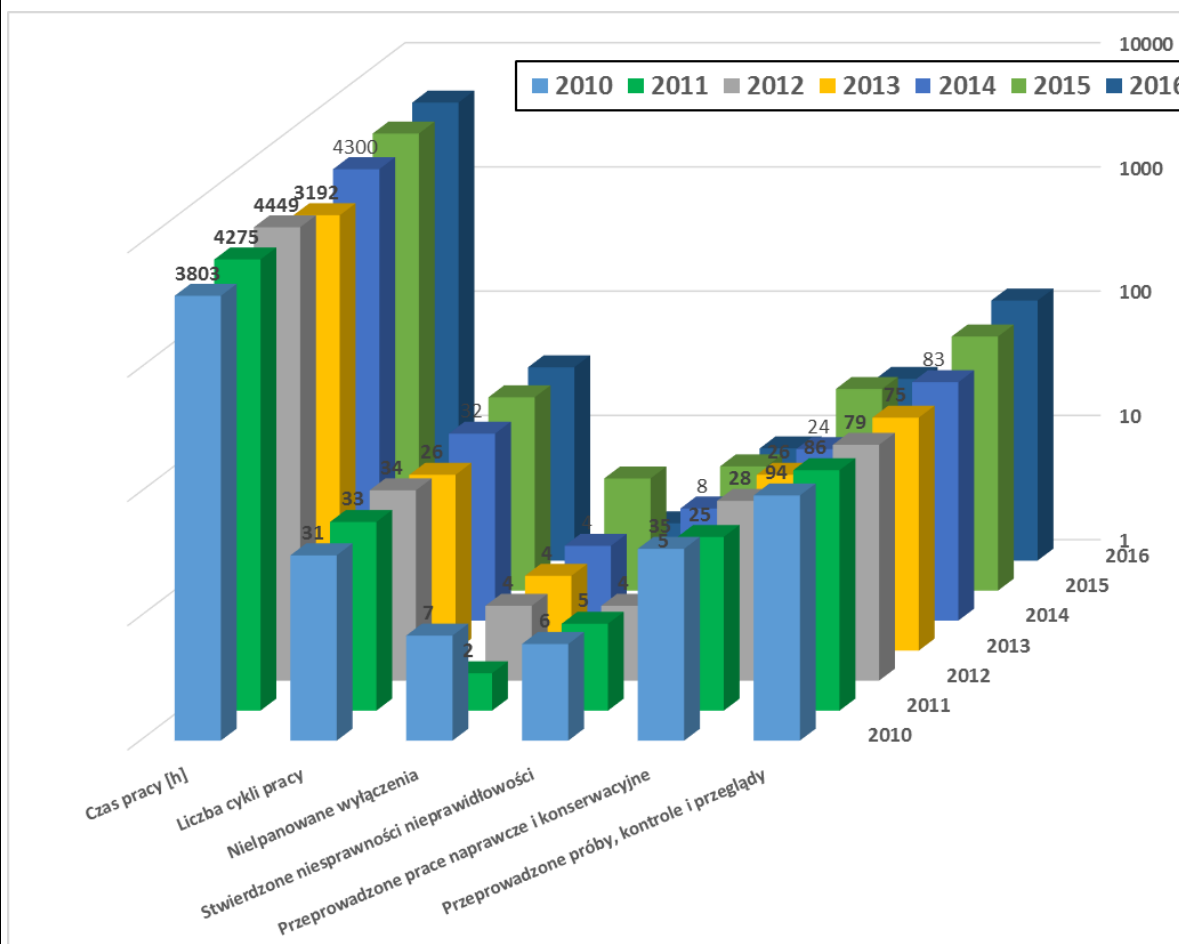
Rysunek 2. Porównanie informacji o eksploatacji reaktora MARIA z ostatnich pięciu lat.
