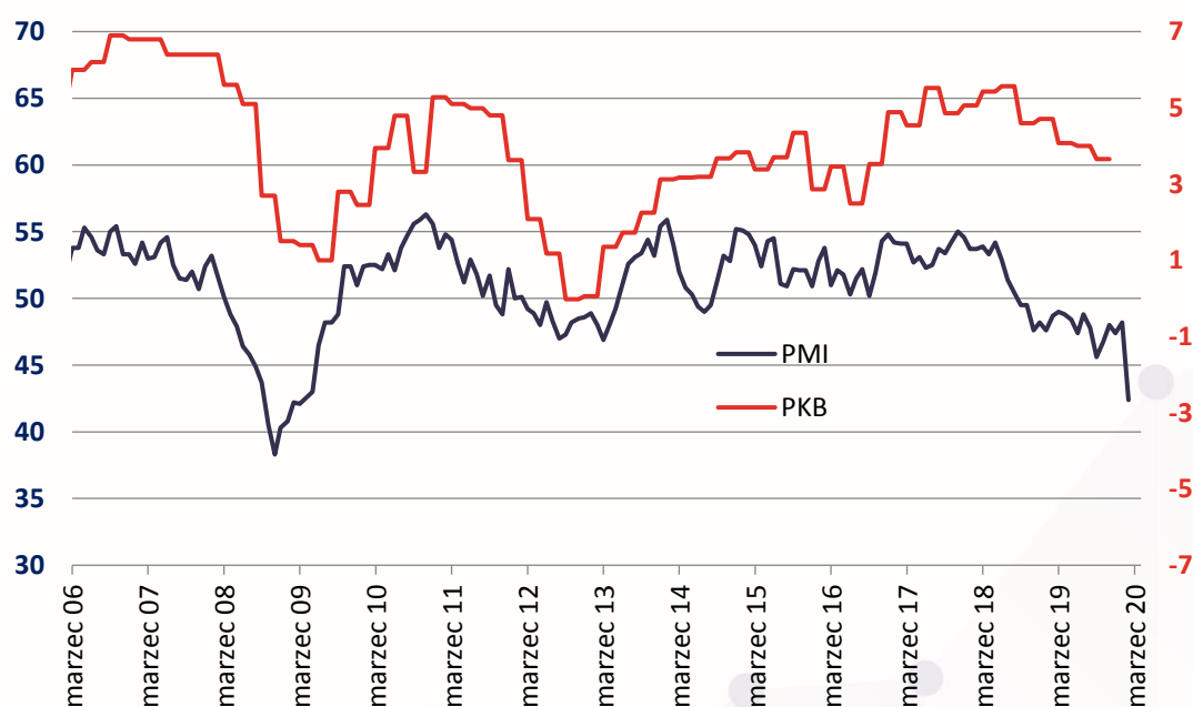
PMI polskiego przemysłu i dynamika PKB rok do roku w kolejnych kwartałach (wyrównana sezonowo)
