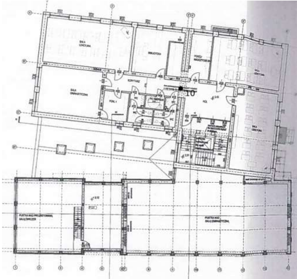
Rys. 1b: Plan rozmieszczenia punktów pomiarowych – 1 piętro
