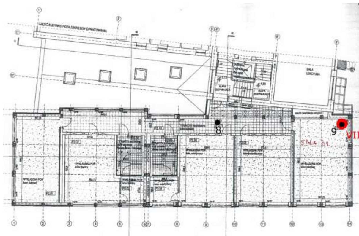
Rys. 1d: Plan rozmieszczenia punktów pomiarowych – nowa część, kolorem czerwonym oznaczono lokalizację punktów dostępowych
