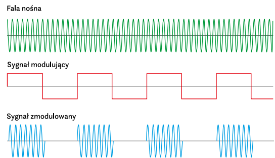
Rys. 5. Cyfrowa modulacja amplitudy. Autor: Paweł Woźniak
