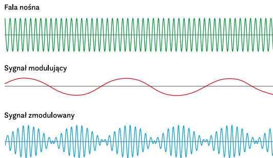
Rys. 4. Analogowa modulacja amplitudy. Autor: Paweł Woźniak
