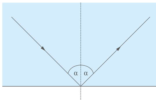
Rys. 2. Zjawisko odbicia fali. Autor: Paweł Woźniak
