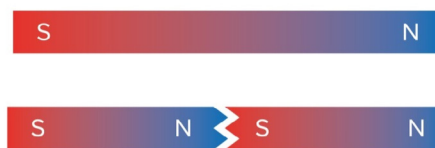
Rys. 4. Podział magnesu sztabkowego. Autor: Paweł Woźniak
