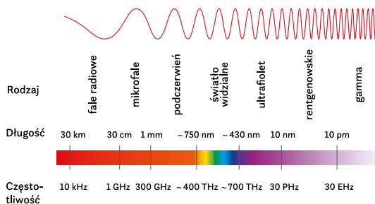
Rys. 3. Widmo fal elektromagnetycznych.
