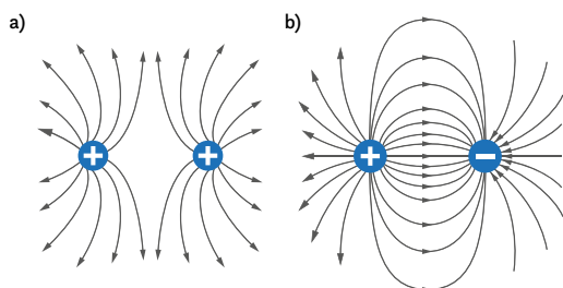
Rys. 2a, b. Linie sił pola elektrycznego wokół ładunków jednoimiennych (a) i różnoimiennych (b). Autor: Paweł Woźniak
