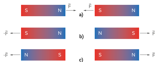
Rys. 5a, b, c. Oddziaływanie biegunów różnoimennych (a) oraz jednoimennych (b, c). Autor: Paweł Woźniak
