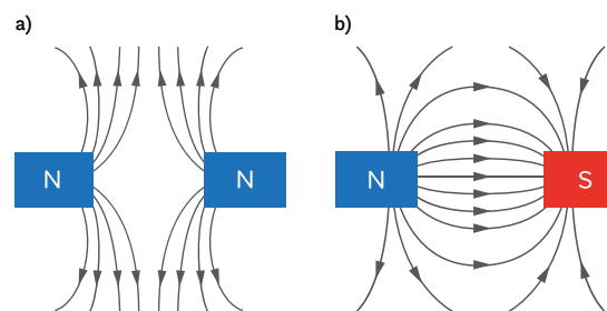
Rys. 6a, b. Linie sił pola magnetycznego wokół biegunów jednoimennych (a) i różnoimennych (b). Autor: Paweł Woźniak
