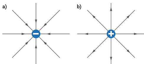
Rys. 1a, b. Linie sił pola elektrycznego wokół pojedynczego punkowego ładunku źródłowego ujemnego (a) i dodatniego (b). Autor: Paweł Woźniak
