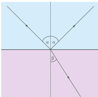
Rys. 4. Zjawisko częściowego załamania i częściowego odbicia fali. Autor: Paweł Woźniak
