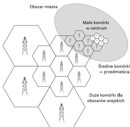
Rys. 3. Pokrycie systemu komórkami według charakterystyki obszaru. Autor: Paweł Woźniak
