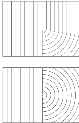
Rys. 5. Zjawisko ugięcia fali. Autor: Paweł Woźniak
