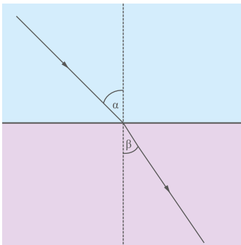
Rys. 3. Zjawisko załamania fali (refrakcji). Autor: Paweł Woźniak
