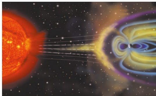
Rys. 2. Wiatr słoneczny i magnetosfera Ziemi. Źródło: Wikimedia Commons
