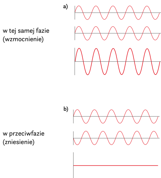
Rys. 6. Zjawisko nakładania się fal w tej samej fazie (a) i różnych fazach (b) – u dołu wypadkowa fala elektromagnetyczna. Autor: Paweł Woźniak
