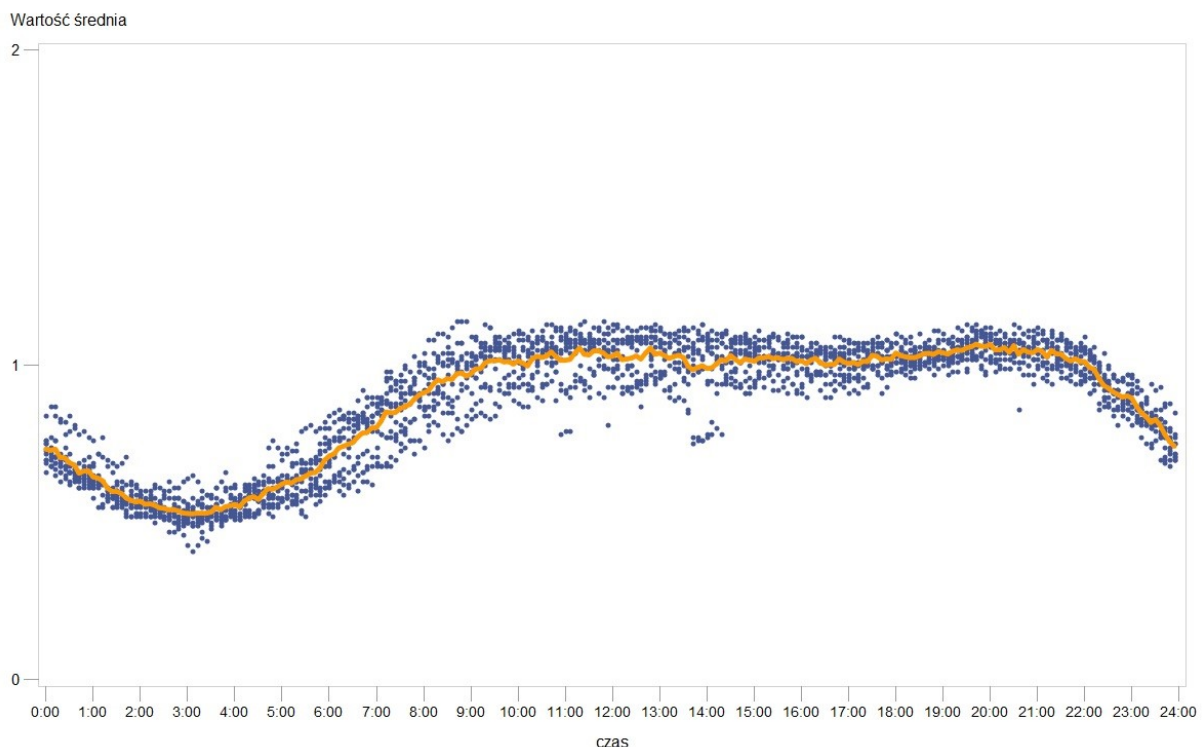
Rys. 8 Wyniki pomiarów – Szkoła Podstawowa nr 1 w Płocku – średnia za okres 24 godzin
