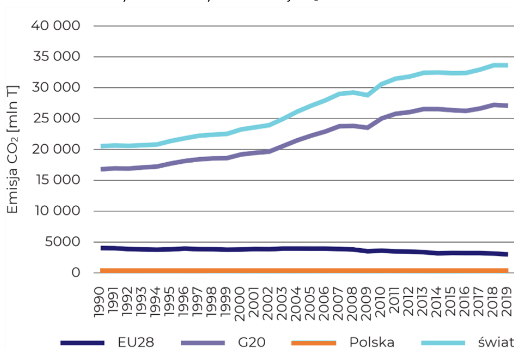
Wykres 12: Zmiany wielkości emisji CO 2 w latach 1990-2019
