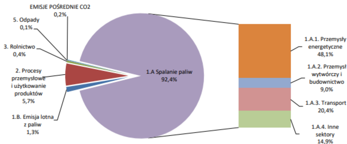
Rysunek 1. Emisja dwutlenku węgla (nieuwzględniająca bilansu emisji netto i pochłaniania CO 2 ) w Polsce w 2021 r. według kategorii źródeł
