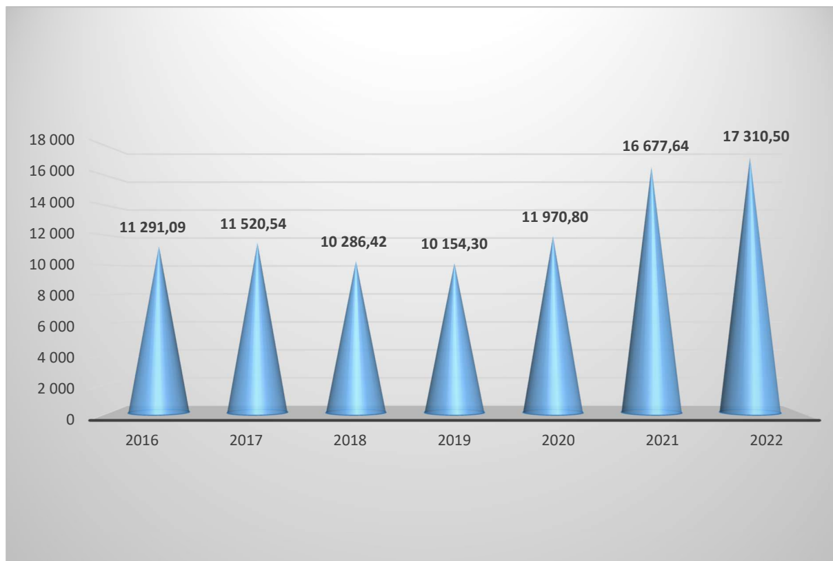
Wykres 6. Wskaźniki efektywności kosztowej PFAZ w latach 2016-2022 (w zł)
