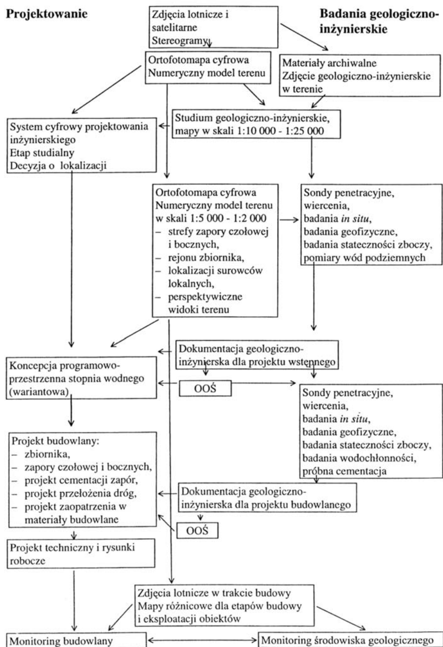
Rys. 9. Schemat organizacji projektowania i badań geologiczno-inżynierskich dla stopnia wodnego
