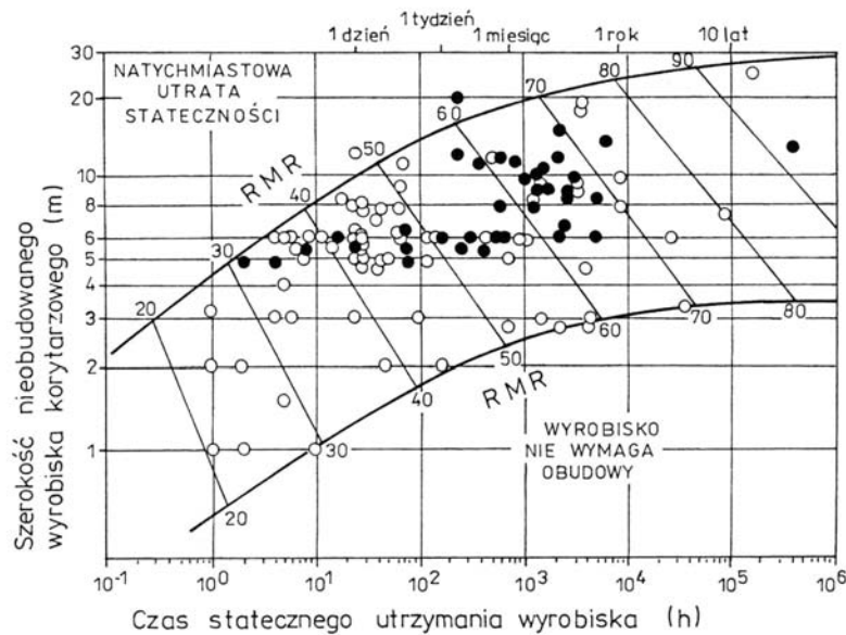
Rys. 13. Zależność między czasem statecznego utrzymania wyrobiska a jego szerokością, w powiązaniu z geomechaniczną klasyfikacją skał wyrażoną wskaźnikiem RMR (wg Z. T. Bieniawskiego)
