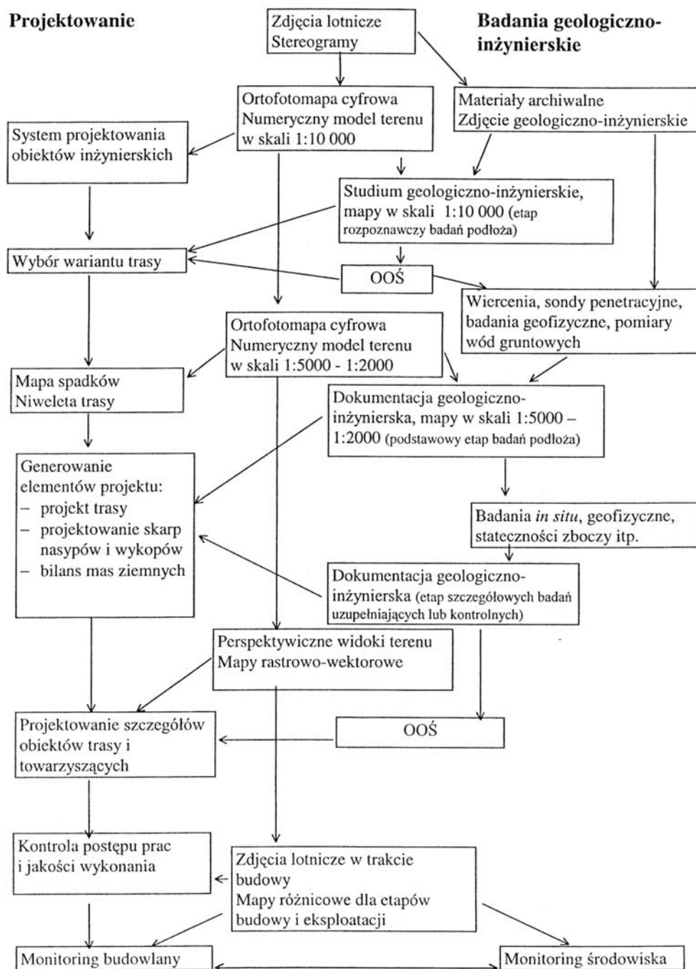
Rys 14. Schemat organizacji projektowania i badań geologiczno-inżynierskich przy budowie autostrady
