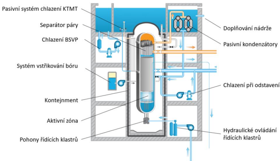
Obr. B.12: Průřez kontejneru BWRX-300
