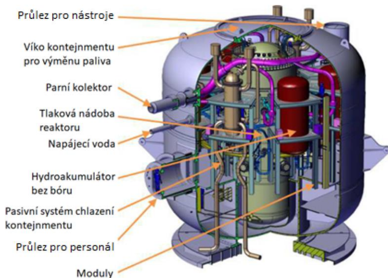
Obr. B.13: Průřez vnitřního kontejneru NUWARD
