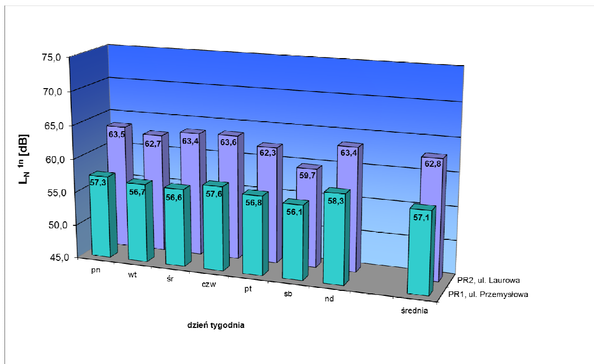
Ryc. 5. Wskaźnik L_N^{1n} (8 h) w [dB]. Zestawienie zmian wskaźnika dla pory nocy ( L_N ) z poszczególnych nocy z 1 tygodniowej sesji pomiarowej wraz z wartością średnią tygodniową, Poczesna 2012 r.
