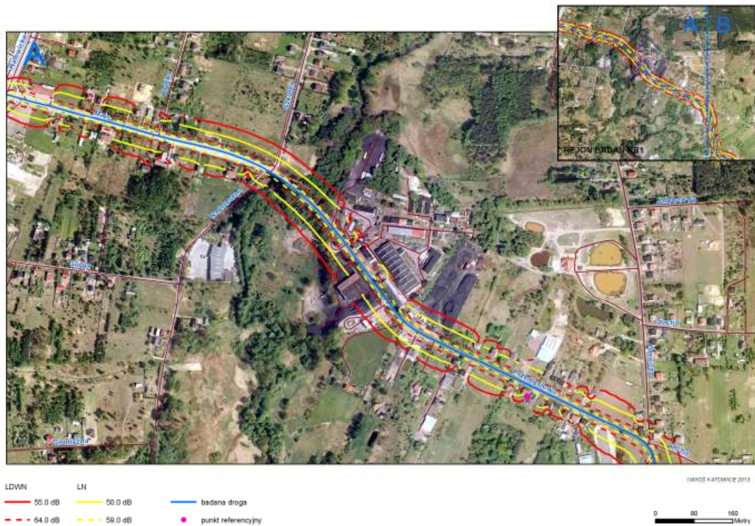
Ryc. 13. Fragment mapy akustycznej „A” dla wskaźnika oceny hałasu L_{DWN} oraz wskaźnika L_N w rejonie badań RB1 – ul. Przemysłowej, Poczesna 2012 rok.
