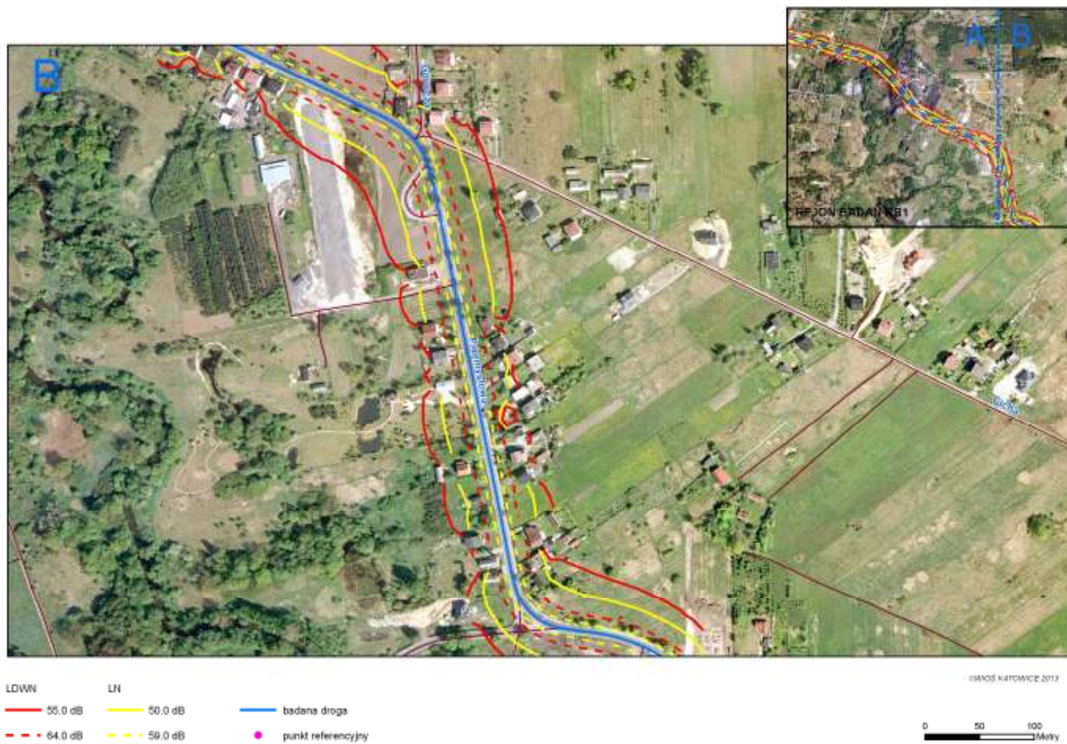
Ryc. 14. Fragment mapy akustycznej „B” dla wskaźnika oceny hałasu L_{DWN} oraz wskaźnika L_N w rejonie badań RB1 – ul. Przemysłowej, Poczesna 2012 rok.
