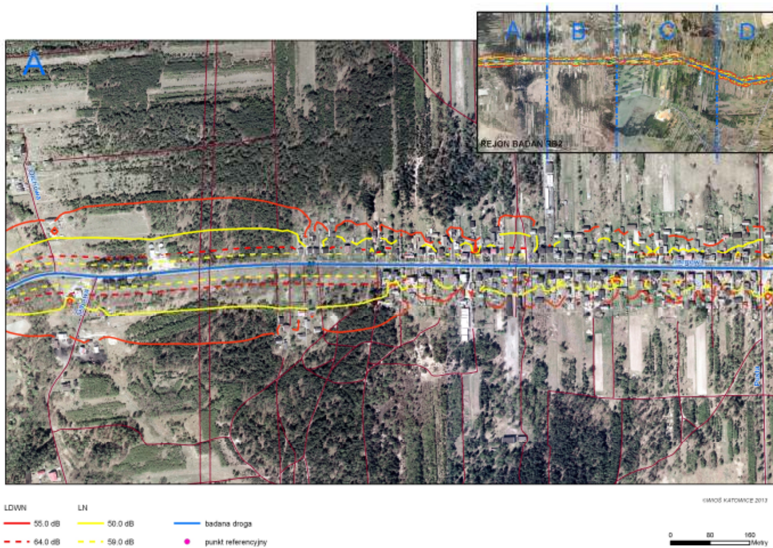
Ryc. 15. Fragment mapy akustycznej „A” dla wskaźnika oceny hałasu L_{DWN} oraz wskaźnika L_N w rejonie badań RB2 – ul. Laurowej, Poczesna 2012 rok.
