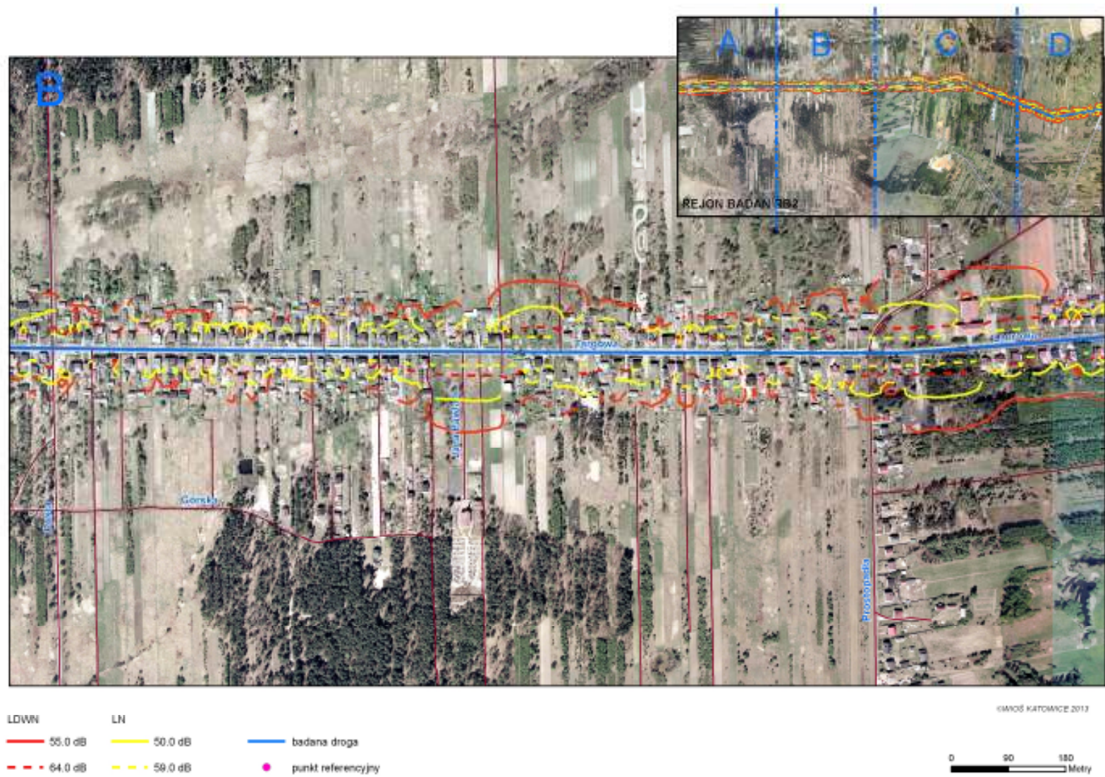
Ryc. 16. Fragment mapy akustycznej „B” dla wskaźnika oceny hałasu L_{DWN} oraz wskaźnika L_N w rejonie badań RB2 – ul. Laurowa, Poczesna 2012 rok.
