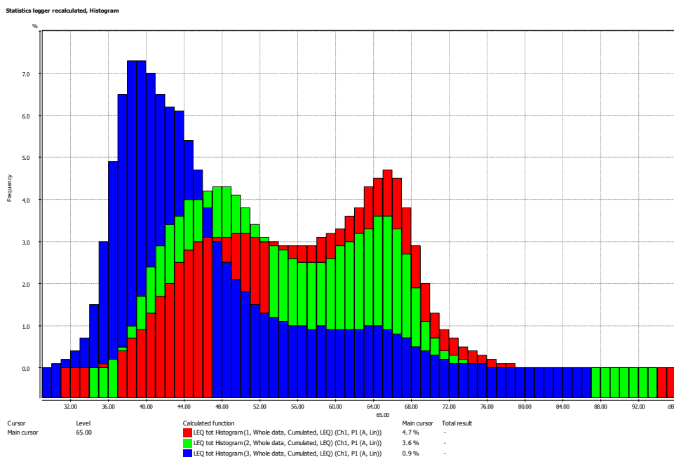
Ryc. 2. Rozkład statystyczny poziomów dźwięku hałasu drogowego dla pory dnia (kol. czerwony), pory wieczoru (kol. zielony) i pory nocy (granatowy) w pkt. pom. PR1 - ul. Przemysłowa, Poczesna, 2012 r. ( z sesji tygodniowej).
