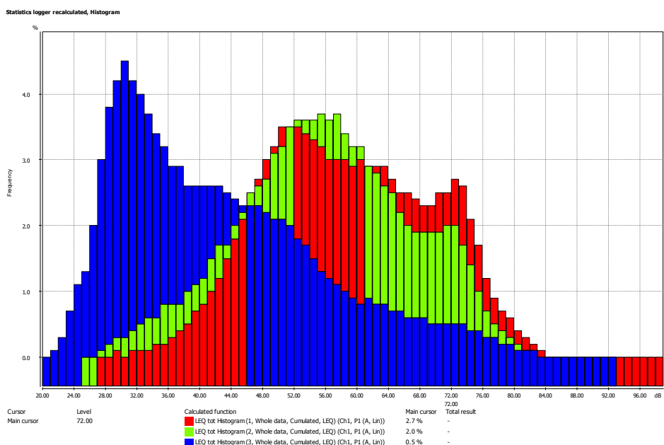
Ryc. 3. Rozkład statystyczny poziomów dźwięku hałasu drogowego dla pory dnia (kol. czerwony), pory wieczoru (kol. zielony) i pory nocy (kol. granatowy) w pkt. pom. PR2 - ul. Laurowa, Poczesna, 2012 r. (z sesji tygodniowej).
