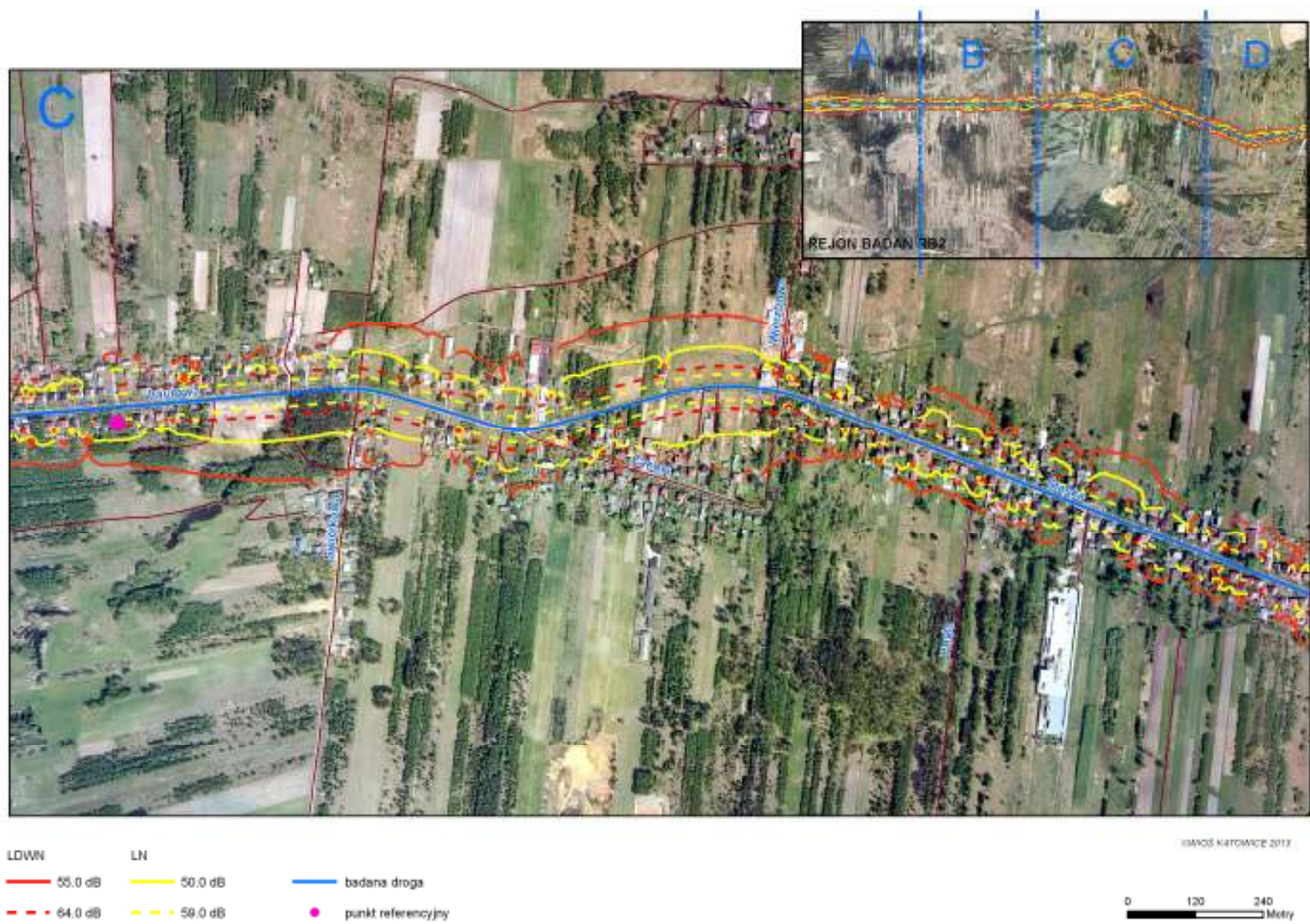
Ryc. 17. Fragment mapy akustycznej „C” dla wskaźnika oceny hałasu L_{DWN} oraz wskaźnika L_N w rejonie badań RB2 – ul. Laurowa, Poczesna 2012 rok.
