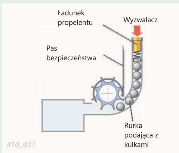
Ilustracja: Schemat zdarzeń podczas aktywacji napinacza
