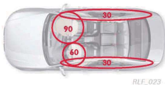
Ilustracja: Strefa zadziałania poduszek powietrznych (cm)
