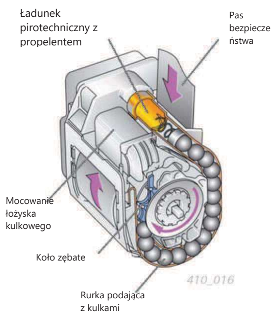
Ilustracja: Przykładowy napinacz z łożyskami kulkowymi
