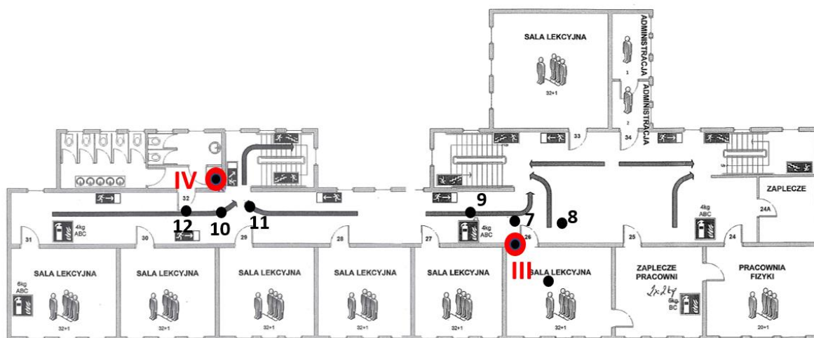
Rys. 1c: Plan rozmieszczenia punktów pomiarowych – II piętro, kolorem czerwonym oznaczono lokalizacje punktów dostępowych
