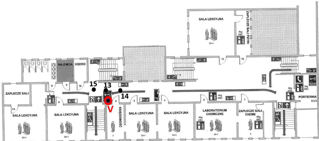
Rys. 1a: Plan rozmieszczenia punktów pomiarowych – parter, kolorem czerwonym oznaczono lokalizację punktów dostępnych
