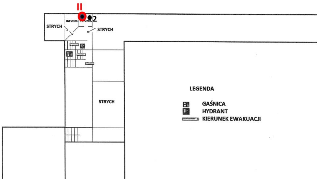
Rys. 1b: Plan rozmieszczenia punktów pomiarowych – strych, kolorem czerwonym oznaczono lokalizację punktów dostępnych
