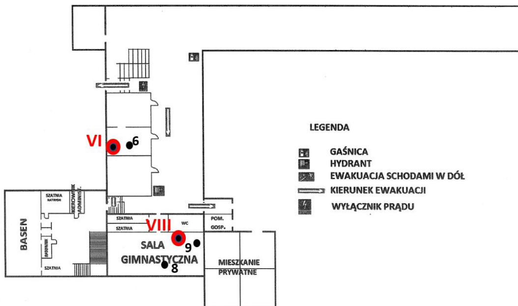
Rys. 1d: Plan rozmieszczenia punktów pomiarowych – parter kolorem czerwonym oznaczono lokalizacje punktów dostępowych
