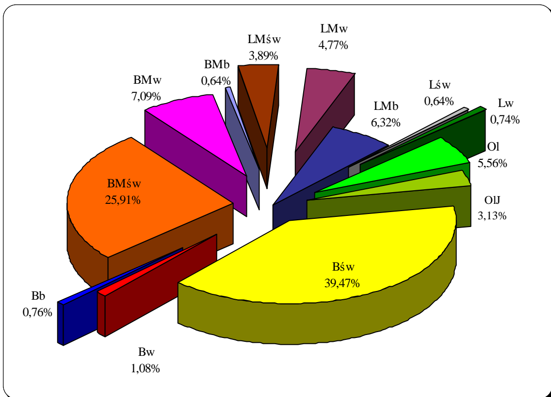
Rycina 10. Udział powierzchni siedliskowych typów lasu w Nadleśnictwie Płaska
