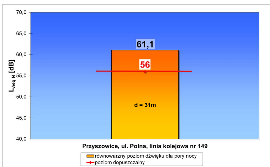
Ryc. 3. Wartość wskaźnika L_{Aeq N} dla rozpatrywanego punktu referencyjnego oraz jego porównanie z obowiązującą wartością poziomu dopuszczalnego, Przyszowice, gmina Gierałtowice, 2022 rok.
