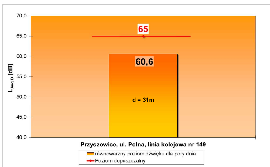
Ryc. 2. Wartość wskaźnika L_{Aeq D} dla rozpatrywanego punktu referencyjnego oraz jego porównanie z obowiązującą wartością poziomu dopuszczalnego, Przyszowice, gmina Gierałtowice, 2022 rok.
