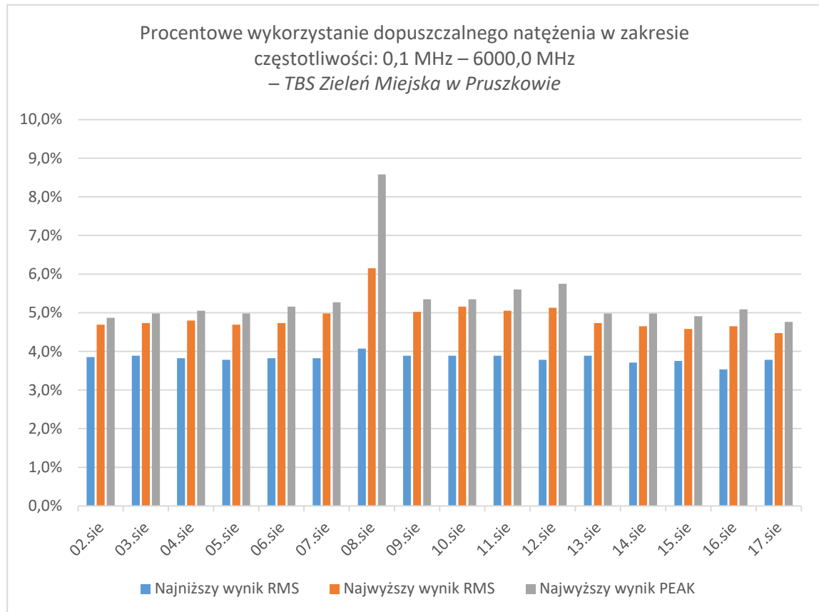
Rys. 26 Procentowe wykorzystanie dopuszczalnego natężenia w zakresie częstotliwości: 0,1 MHz – 6000,0 MHz – TBS Zieleń Miejska w Pruszkowie
