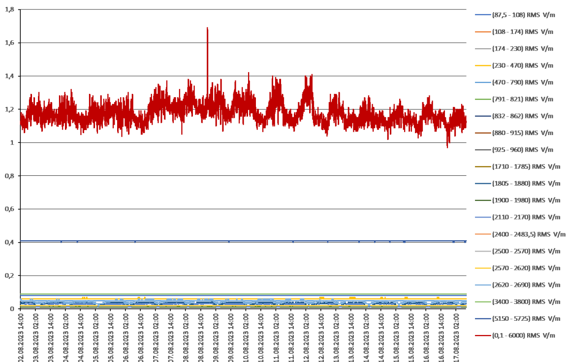
Rys. 5 Wyniki pomiarów dla 20 podzakresów częstotliwości – TBS Zieleń Miejska w Pruszkowie
