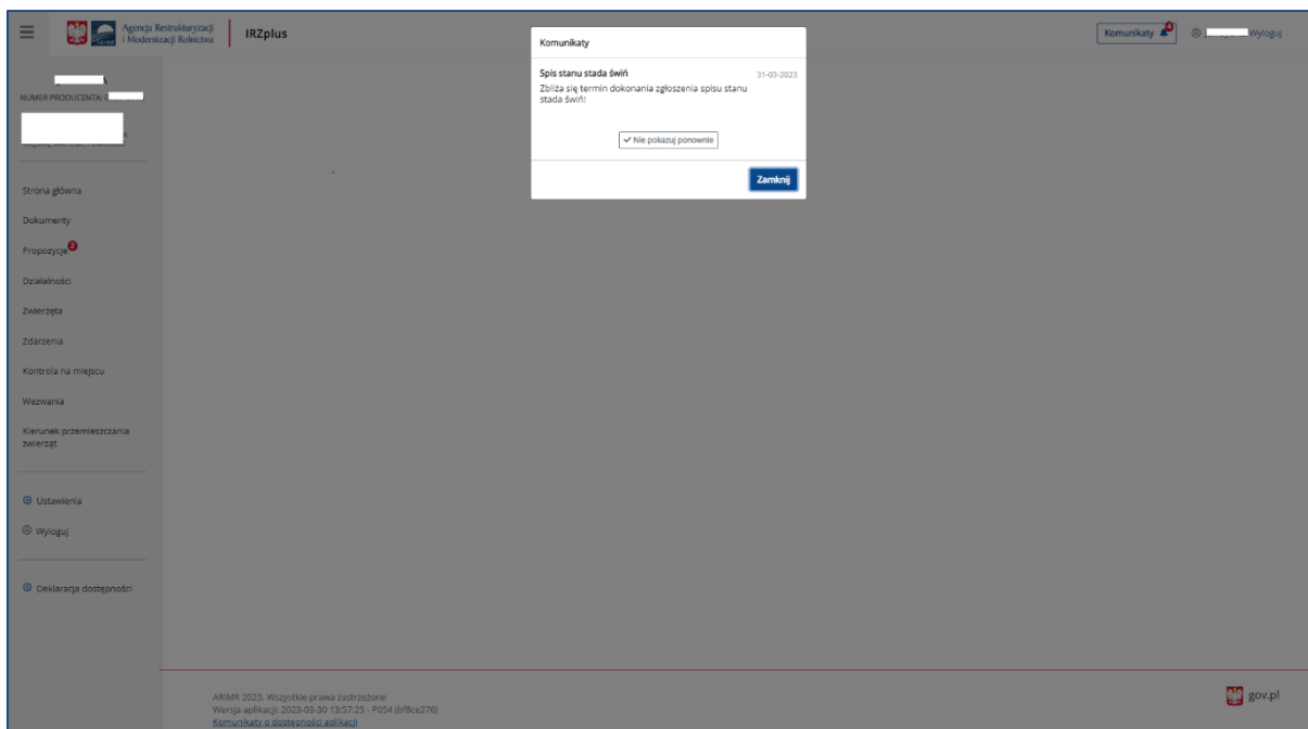
Rysunek 10 Komunikaty
