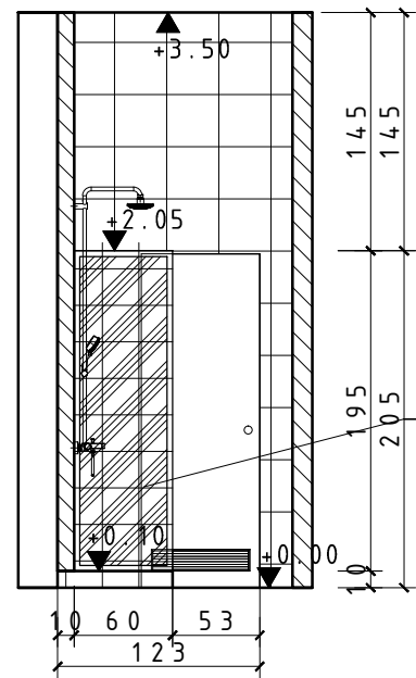
PRZEKRÓJ A-A
