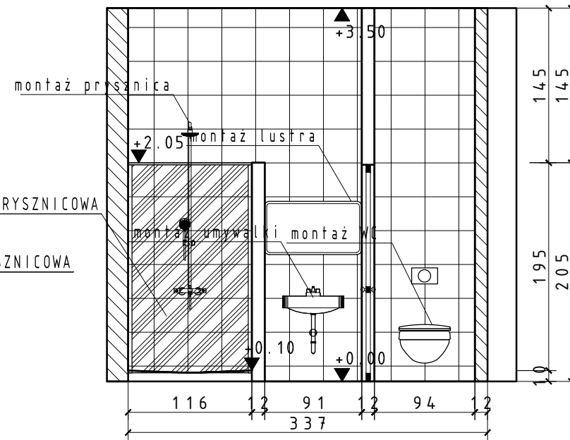
PRZEKRÓJ B-B
