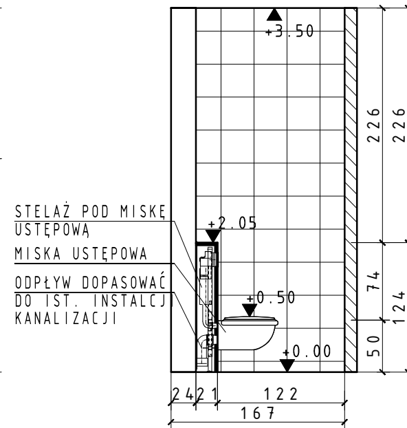
PRZEKRÓJ D-D
