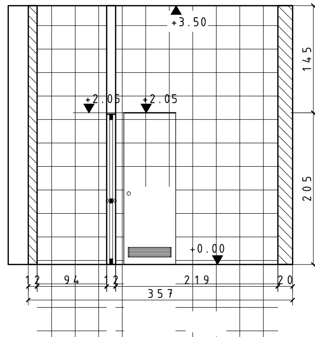
PRZEKRÓJ C-C
