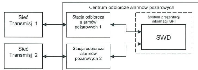
Rys. 3. Schemat systemu transmisji alarmów pożarowych bez stacji koncentracji.
