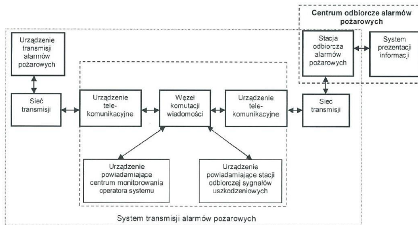
Rys. 2. System transmisji alarmów pożarowych ze stacją pośredniczącą
