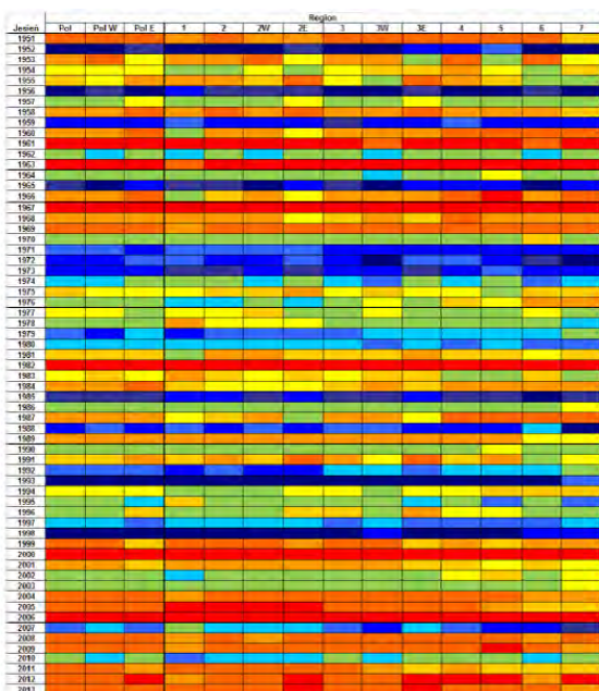
Rys. 7.29. Klasyfikacja temperatury powietrza w sezonach jesiennych
