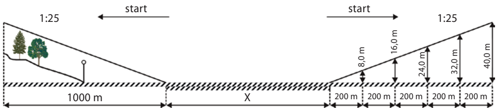
Rycina 2. Przekrój podłużny pasa startowego
