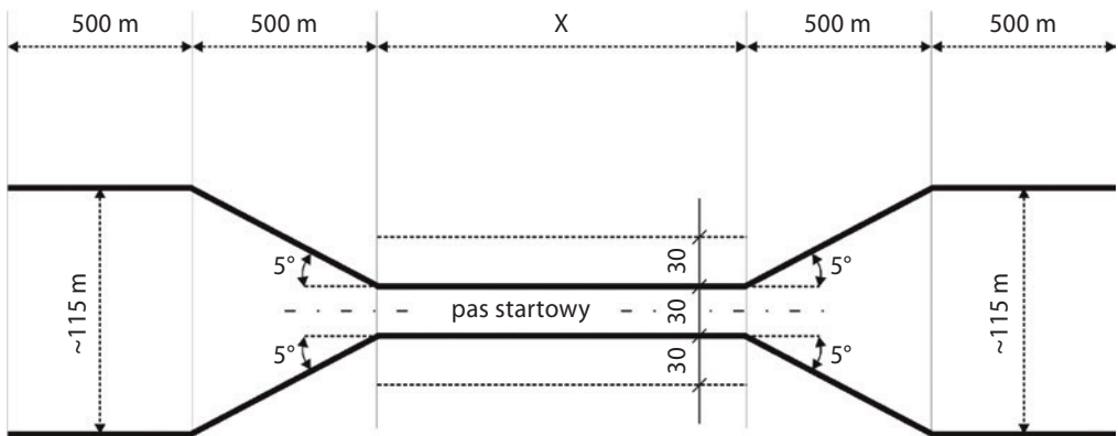
Rycina 1. Rzut poziomy pasa startowego
