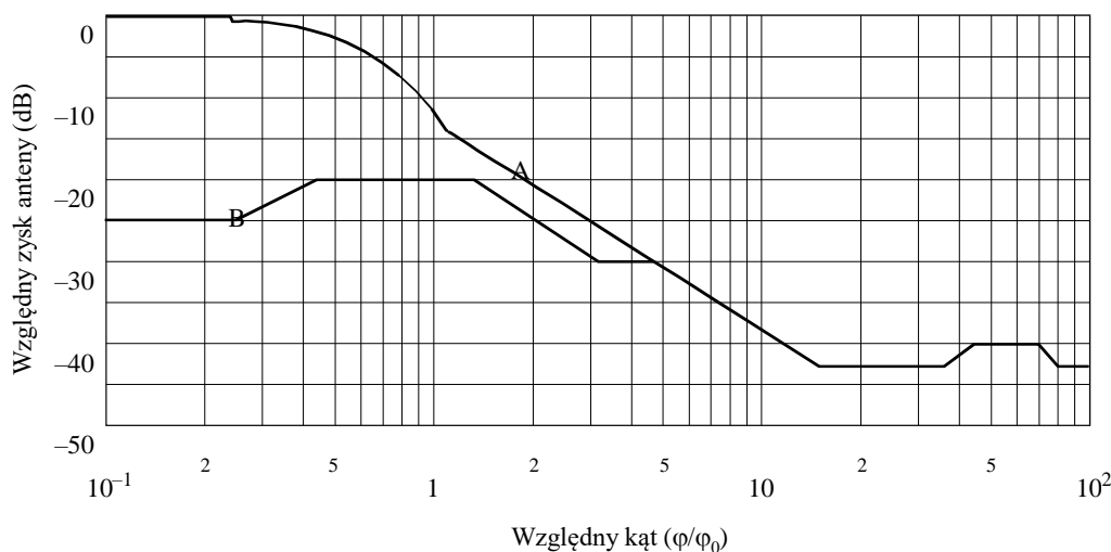
Rysunek 8 Charakterystyki odniesienia w przypadku składowych o polaryzacjach zgodnych i ortogonalnych w odniesieniu do anten stacji ziemskich w Regionie 2
