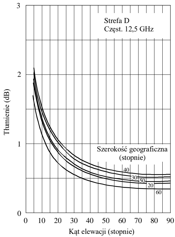
d) Deszczowa strefa klimatyczna D
