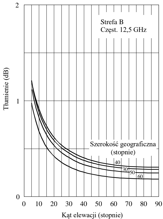
b) Deszczowa strefa klimatyczna B
