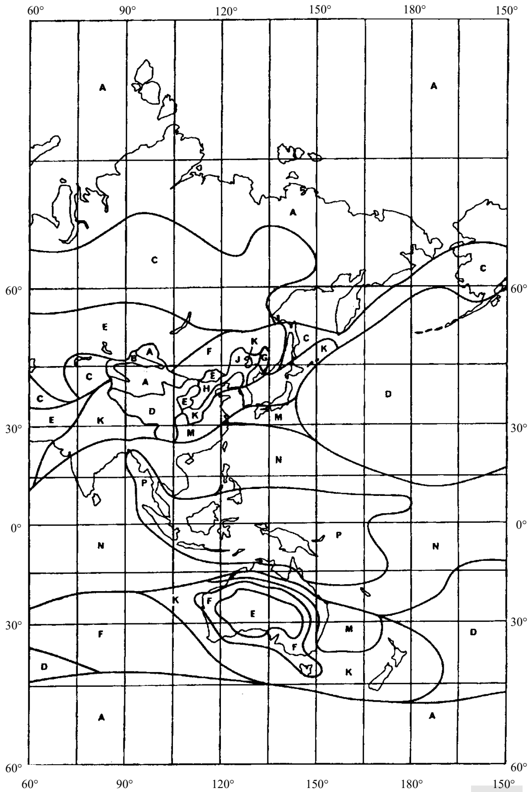
Deszczowe strefy klimatyczne dla Regionów 1 i 3 między długościami geograficznymi 60° E i 150° W
