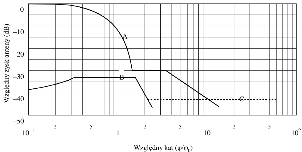
Rysunek 9 Charakterystyki odniesienia dla składowych o polaryzacjach zgodnych nadawczej anteny satelitarnej w Regionach 1 i 3
