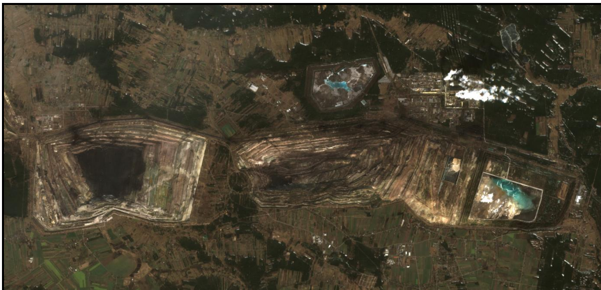
Ryc. 4.10-3 Kopalnia węgla brunatnego i elektrownia, Bełchatów, zobrazowanie satelitarne Sentinel-2, III 2021. 252
