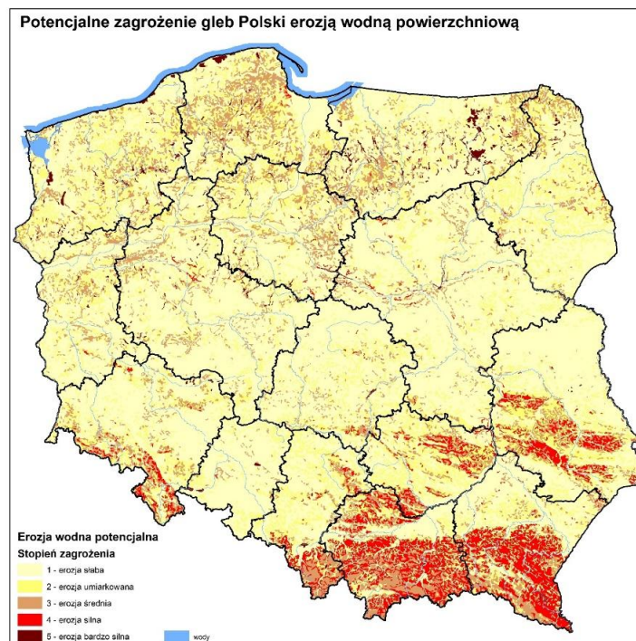
Ryc. 4.7-17 Mapa zagrożenia gleb erozją wodną powierzchniową w Polsce. 215
