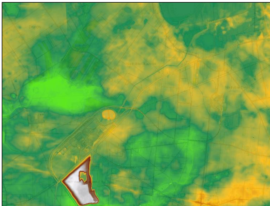
Ryc. 4.10-2 Okolice KW Bogdanka, widoczne deformacje terenu na Modelu Wysokościowym Terenu utworzonym z wykorzystaniem technologii lotniczego skaningu laserowego. 250
