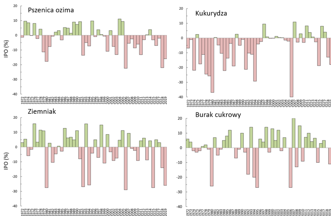
Ryc. 5.1-1 Wskaźnik pogodowy plonu krajowego (IPO) pszenicy ozimej, kukurydzy, ziemniaka i buraka cukrowego w latach 1972-2019. (Źródło: Kozyra i inni., 2012, uzupełnione). 301
