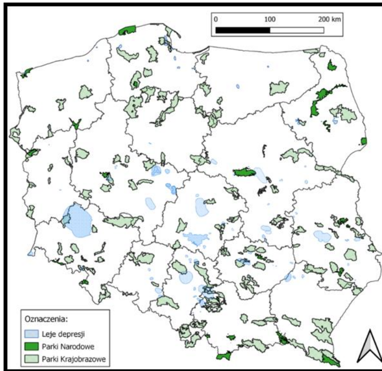
Ryc. 4.5-5. Lokalizacja lejów depresji na tle Parków Narodowych i Parków Krajobrazowych źródło: Opracowanie własne na podstawie danych z Generalnej Dyrekcji Ochrony Środowiska.
