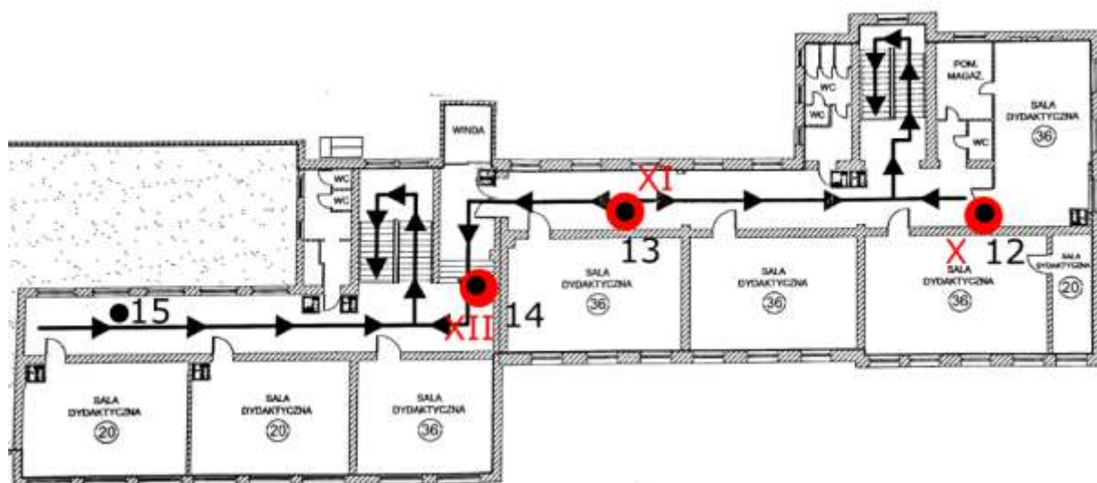
Rys. 1c: Plan rozmieszczenia punktów pomiarowych – II piętro, kolorem czerwonym oznaczono lokalizację punktów dostępnych
