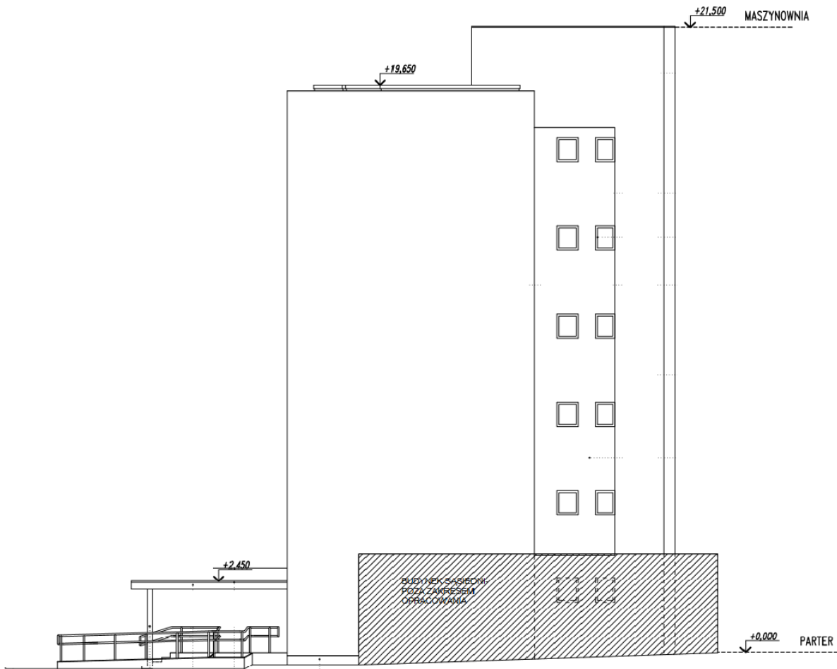
Elewacja zachodnia ul. Lisa Kuli 20
