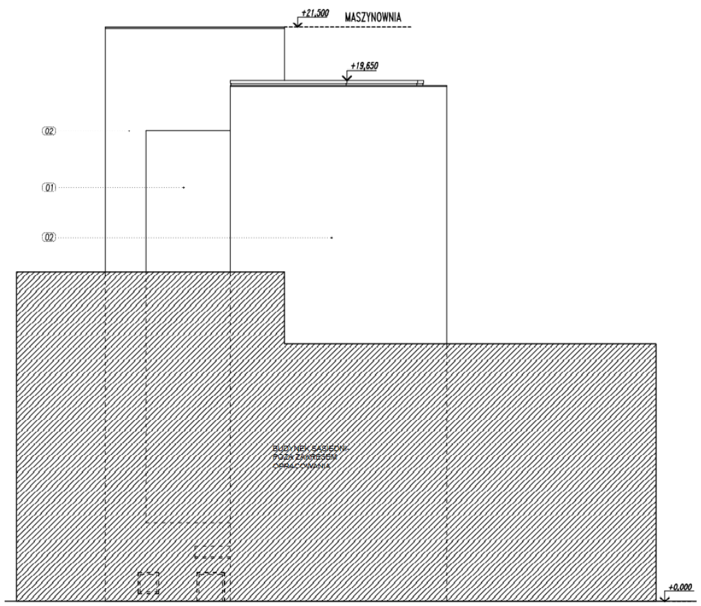
Elewacja wschodnia ul.Lisa Kuli 20
