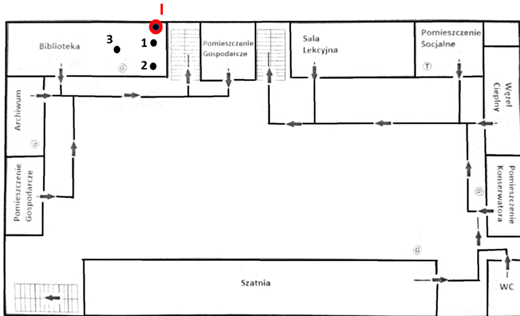
Rys. 1a: Plan rozmieszczenia punktów pomiarowych – Piwnica, kolorem czerwonym oznaczono lokalizację punktów dostępnych
