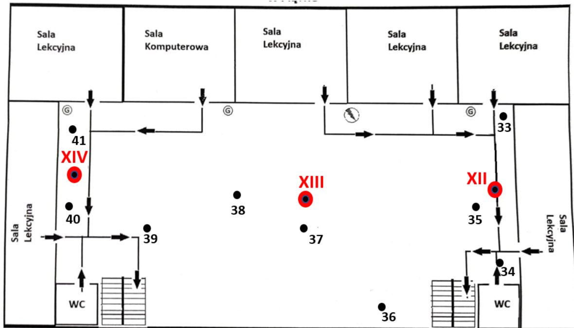
Legenda: Rys. 1e: Plan rozmieszczenia punktów pomiarowych – III Piętro, kolorem czerwonym oznaczono lokalizację punktów dostępowych
