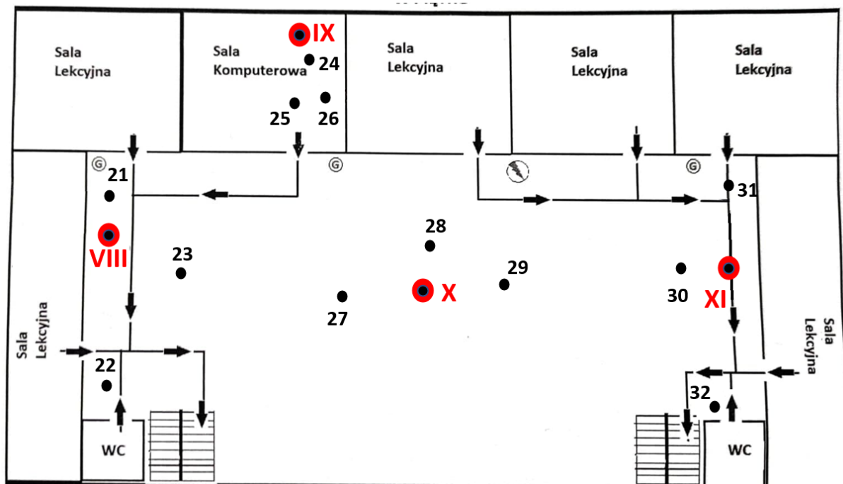
Rys. 1d: Plan rozmieszczenia punktów pomiarowych – II Piętro, kolorem czerwonym oznaczono lokalizację punktów dostępowych
