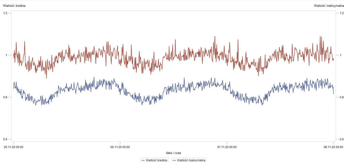
Rys. 6 Wyniki pomiarów – UM Białystok w okresie 5.11.2020 r. – 8.11.2020 r.
