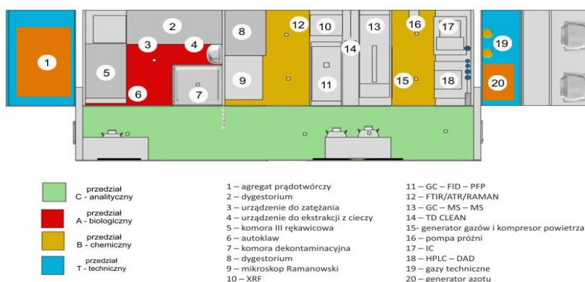
KONCEPCJA ZABUDOWY SAMOCHODU LABORATORIUM DLA WIODĄCYCH GRUP RADIACJI - BILOGII
