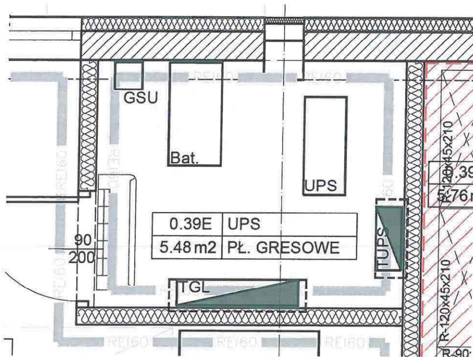
Rys. 2. Rysunek poglądowy z przykładowym rozmieszczeniem zasilacza awaryjnego UPS
