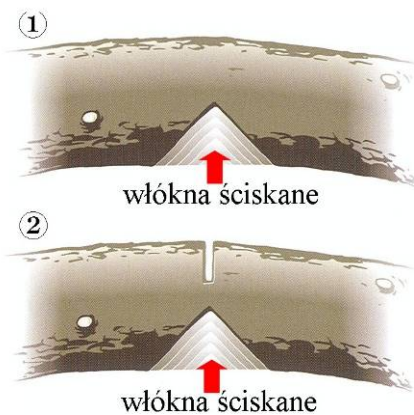
Rys.69 Cięcie drewna o dużych naprężeniach – rzał w kształcie litery „V”.
