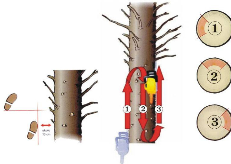
Rys.43 Wahadłowa technika okrzyszwania drzew.
