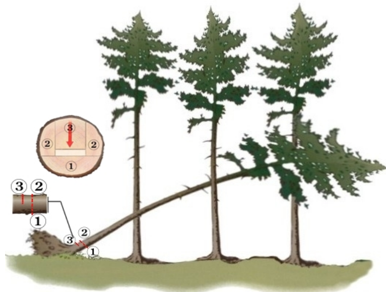
Rys.66 Kolejność i przesunięcie rżazów przy cięciu drewna o większych naprężeniach na przykładzie odcinania bryły korzeniowej wywrotów pochylonych, wplecionych między drzewa stojące.
