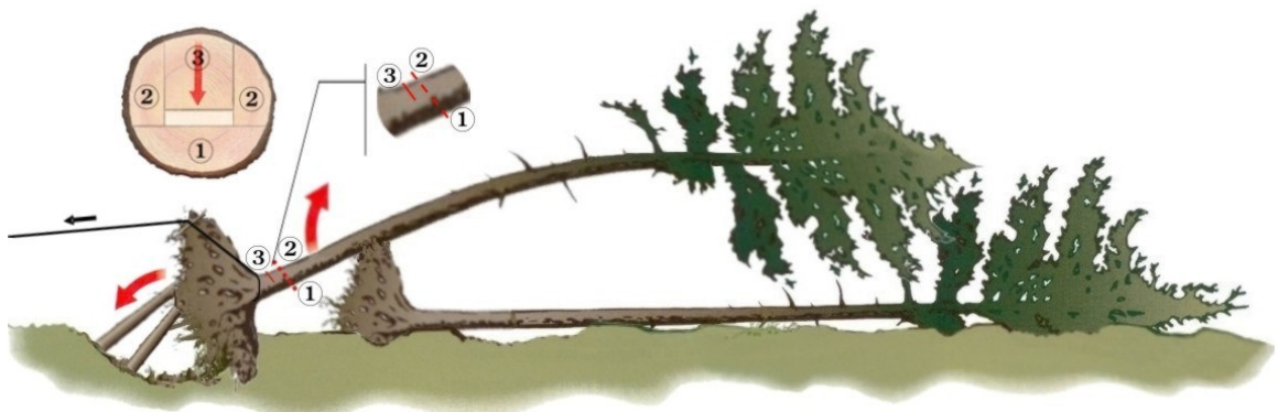
Rys.65 Kolejność i przesunięcie rżazów przy cięciu drewna o większych naprężeniach na przykładzie odcinania bryły korzeniowej wywrotów wspartych na strzałach lub bryłach korzeniowych innych drzew, ze środkiem ciężkości za podporą.
