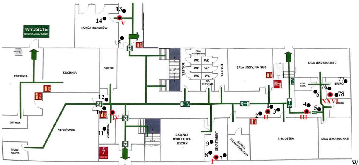
Rys. 1h Plan rozmieszczenia punktów pomiarowych – parter kolorem czerwonym oznaczono lokalizację punktów dostępnych
