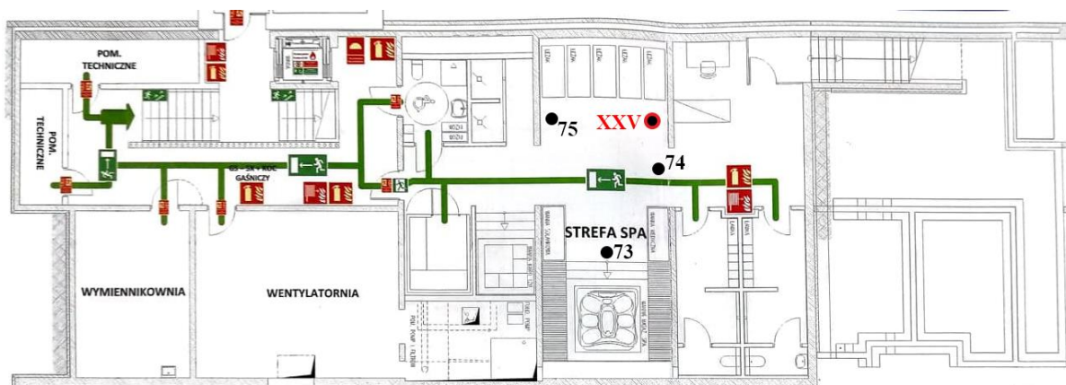
Rys. 1i Plan rozmieszczenia punktów pomiarowych – parter kolorem czerwonym oznaczono lokalizację punktów dostępowych
