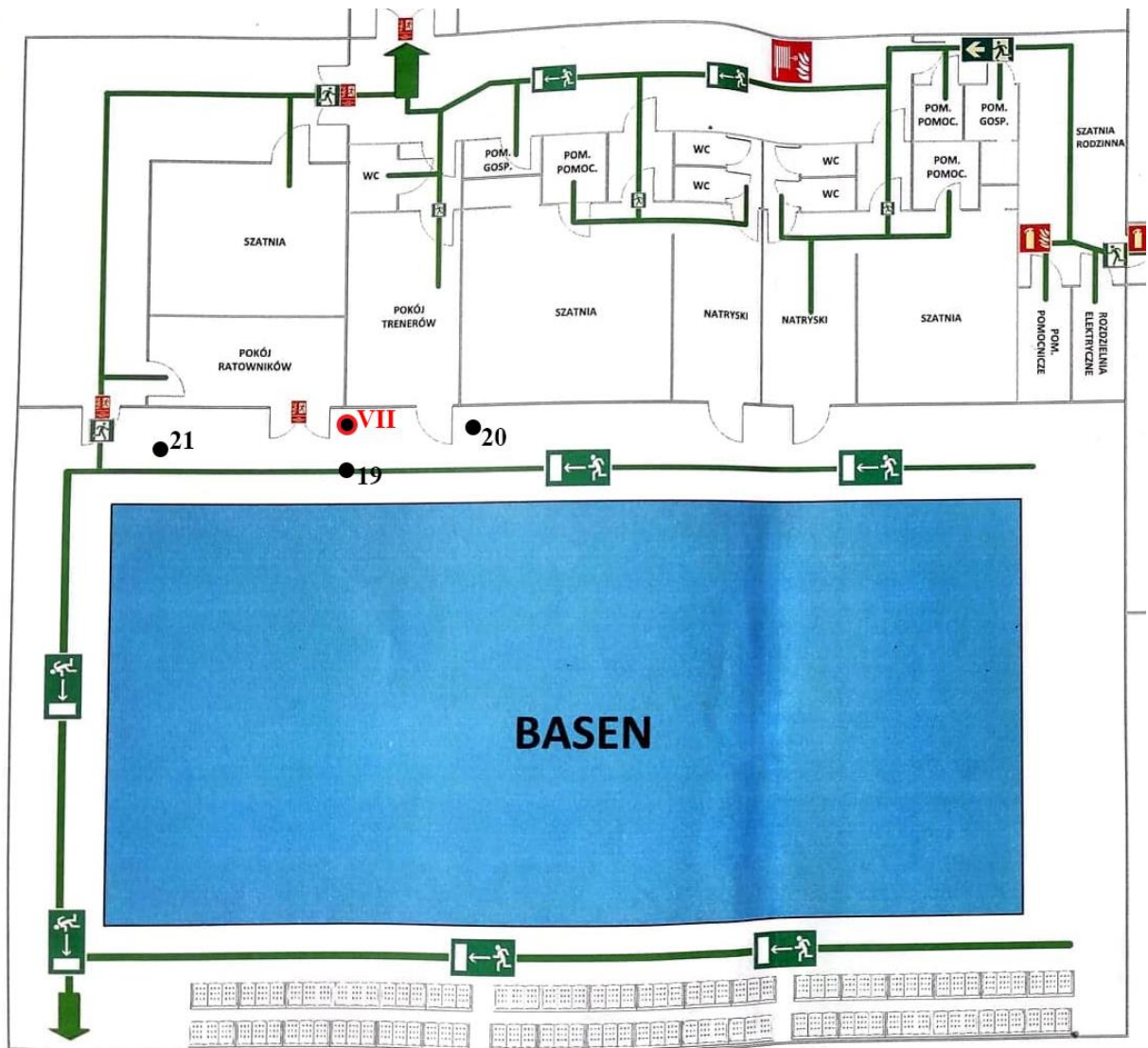
Rys. 1f: Plan rozmieszczenia punktów pomiarowych – basen kolorem czerwonym oznaczono lokalizację punktów dostępnych
