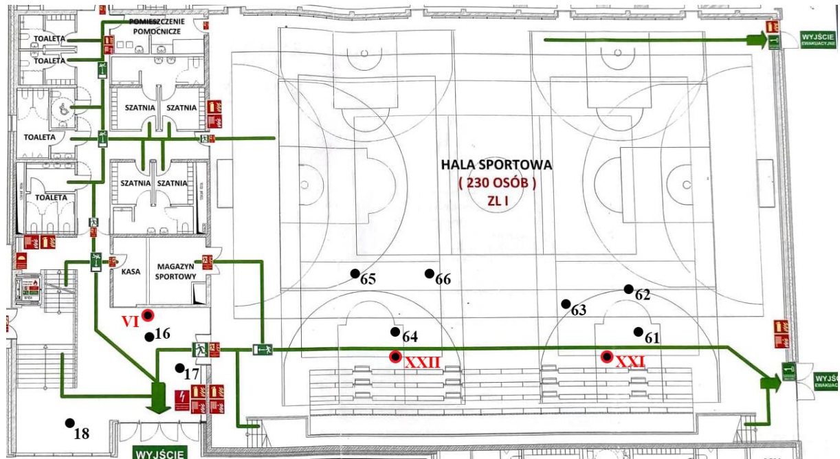
Rys. 1g Plan rozmieszczenia punktów pomiarowych – hala sportowa kolorem czerwonym oznaczono lokalizację punktów dostępnych
