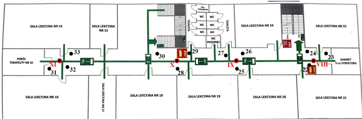
Rys. 1a: Plan rozmieszczenia punktów pomiarowych – 1 piętro, kolorem czerwonym oznaczono lokalizację punktów dostępowych
