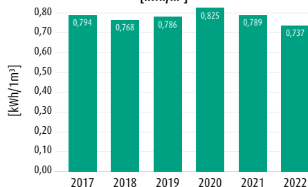
Zużycie energii elektrycznej na ujęcie i wtłoczenie 1m 3 wody, z UW Wierchowisko do sieci wodociągowej w latach 2017 - 2022 [kWh/m 3 ]
