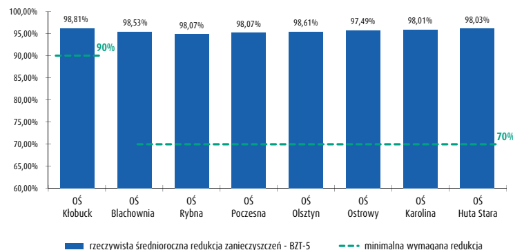
Średnioroczne wartości redukcji zanieczyszczeń wskaźnika BZT-5 w oczyszczalniach ścieków w 2022r. [%]
