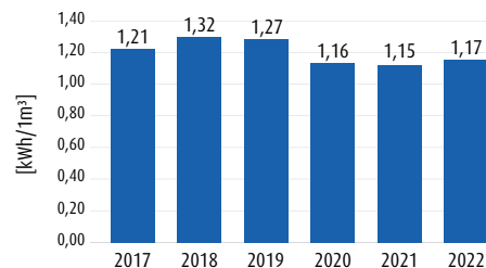
Zużycie energii elektrycznej na oczyszczenie 1 m 3 ścieków komunalnych w oczyszczalni ścieków w Kłobucku w latach 2017 - 2022 [kWh/m 3 oczyszczonych ścieków]
