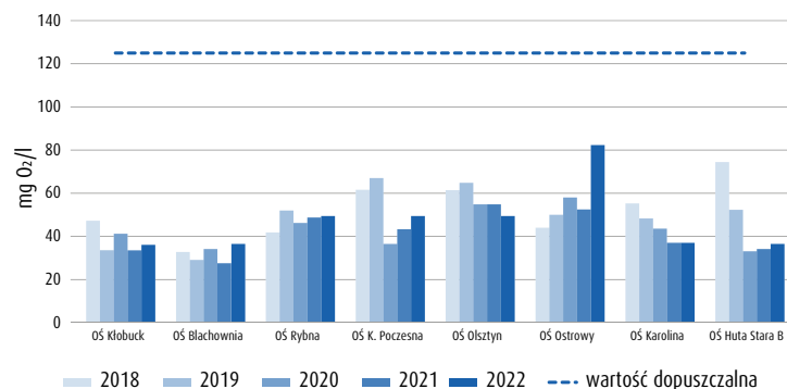
Średnioroczne stężenie wskaźnika „ChZT” w ściekach oczyszczonych odprowadzanych z poszczególnych oczyszczalni ścieków do odbiornika w latach 2018 – 2022
