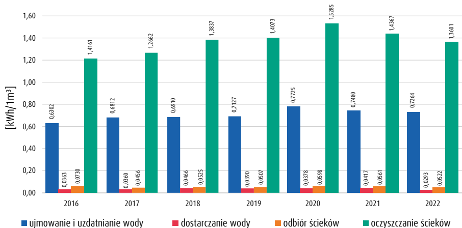
Jednostkowe zużycie energii elektrycznej na procesy: ujmowania i uzdatniania wody, dostarczenia wody, odbioru i oczyszczania ścieków w latach 2016 - 2022 [ kWh/1m 3 ]
