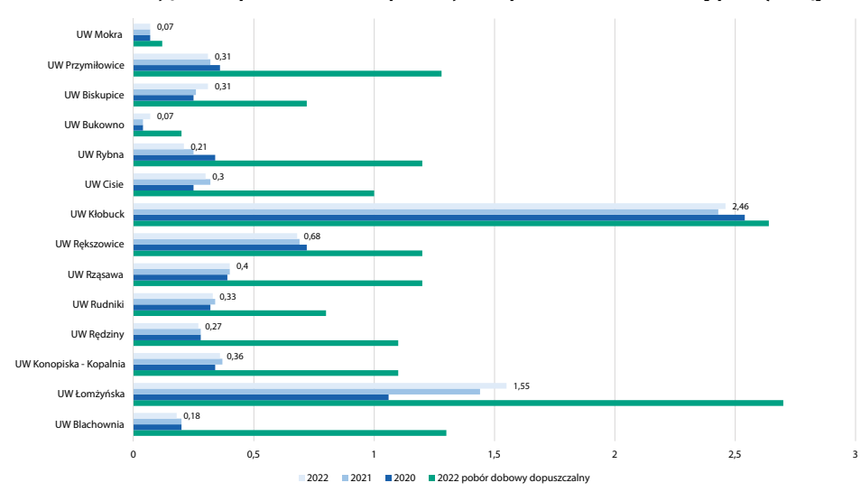
Pomocnicze ujęcia wody. Średniodobowa produkcja wody w latach 2020 - 2022 [tys. m 3 /dobę]
