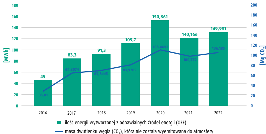
Ilość energii elektrycznej wytworzonej z odnawialnych źródeł energii (OZE) [MWh] oraz wielkość pomniejszenia emisji dwutlenku węgla do atmosfery [MgCO 2 ] w latach 2016 – 2022
