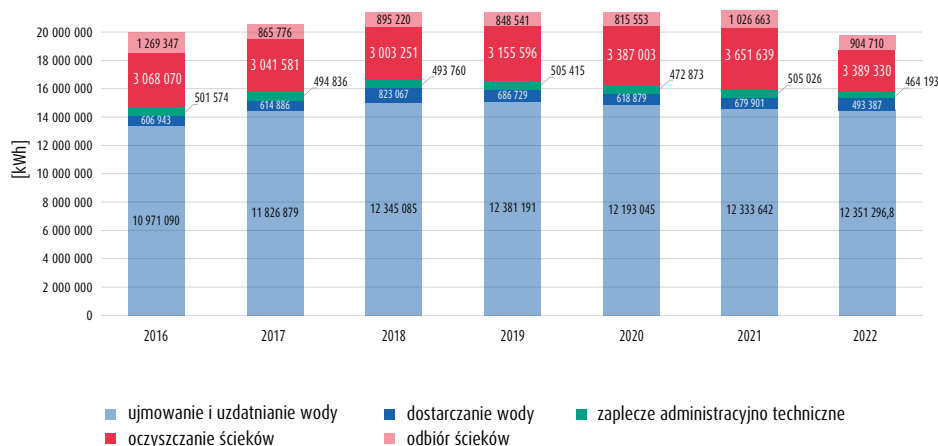
Zużycie energii elektrycznej na procesy: ujmowania i uzdatniania wody, dostarczania wody oraz odbioru i oczyszczania ścieków w latach 2016 - 2022 [ kWh/rok]
