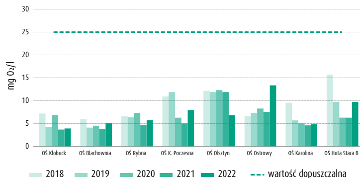
Średnioroczne stężenia wskaźnika BZT 5 w ściekach oczyszczonych odprowadzanych z poszczególnych oczyszczalni ścieków do odbiornika w latach 2018 – 2022
