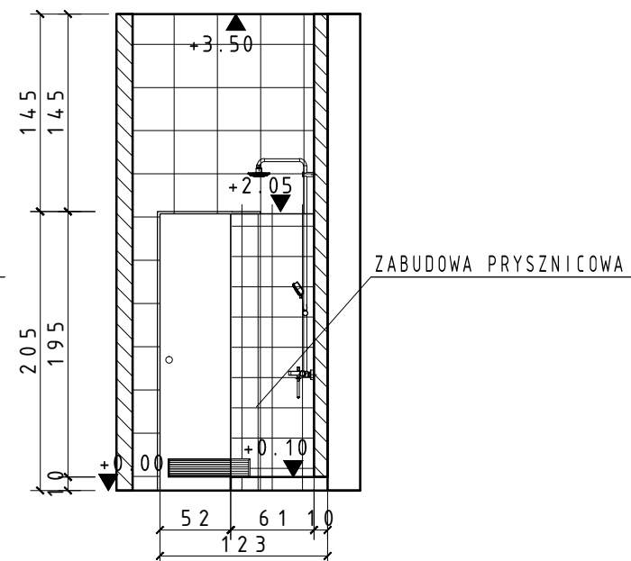
PRZEKRÓJ D-D
