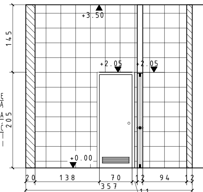
PRZEKRÓJ B-B
