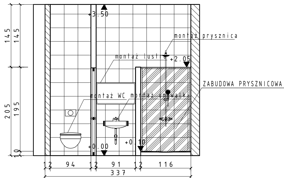
PRZEKRÓJ C-C
