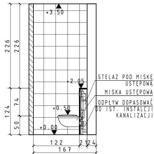
PRZEKRÓJ A-A
