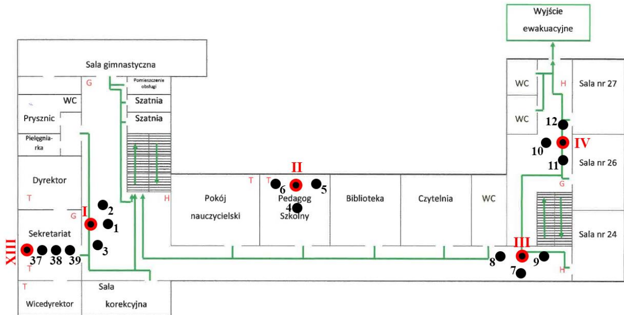
Rys. 1a: Plan rozmieszczenia punktów pomiarowych – I Piętro, kolorem czerwonym oznaczono lokalizację punktów dostępowych
