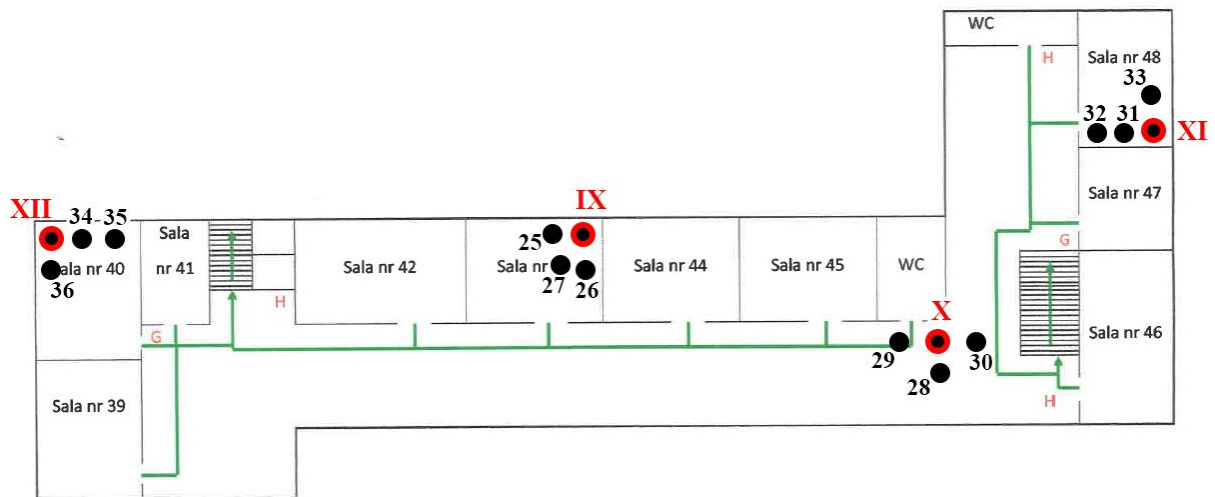
Rys. 1c: Plan rozmięszczenia punktów pomiarowych – III Piętro, kolorem czerwonym oznaczono lokalizację punktów dostępowych
