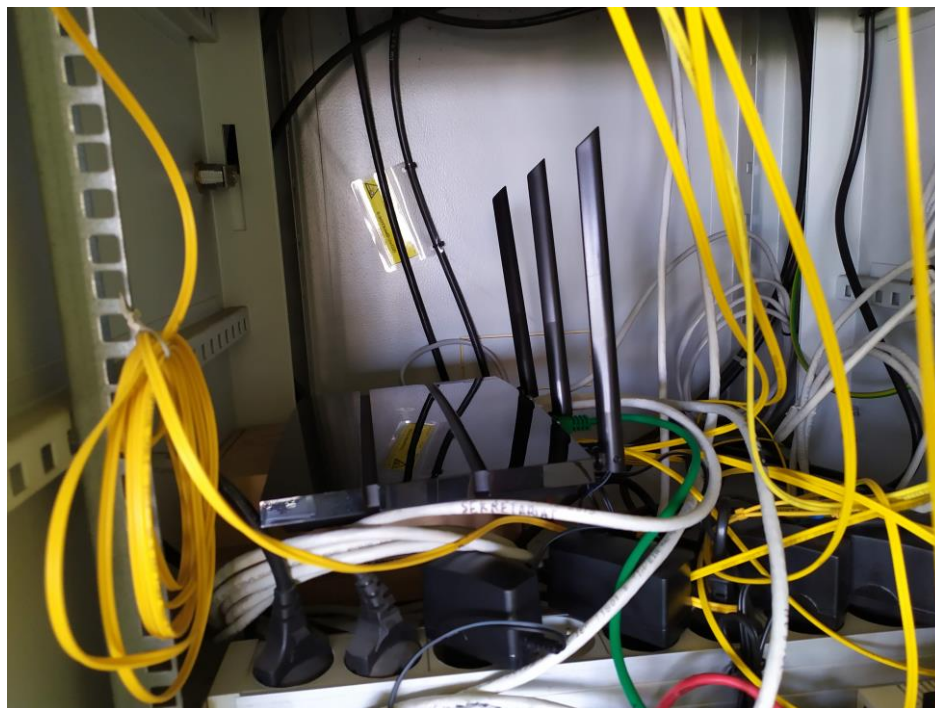
Fot. 2: Punkt dostępowy model TP-LINK Archer C1200
