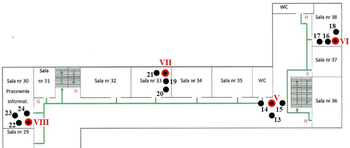
Rys. 1b: Plan rozmieszczenia punktów pomiarowych – II Piętro, kolorem czerwonym oznaczono lokalizację punktów dostępowych
