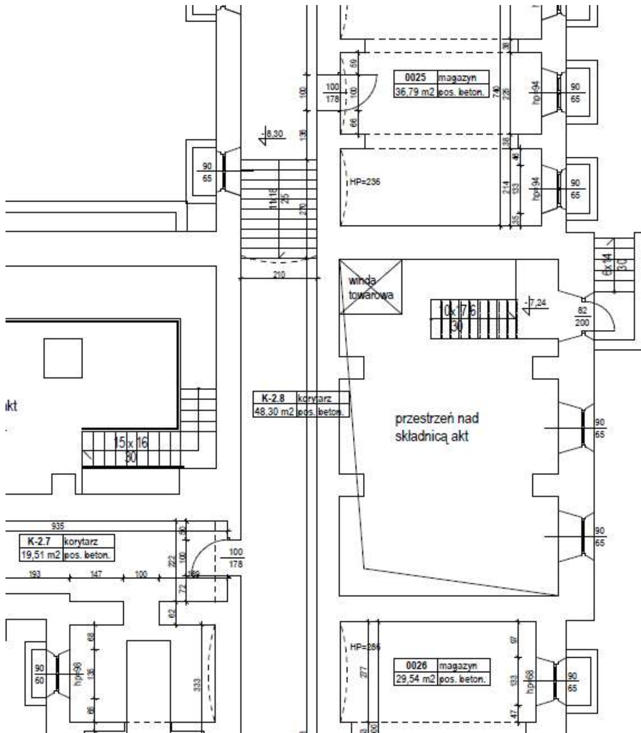
Rys. Nr 3 Fragment rzutu piwnicy – Składnica Akt.
