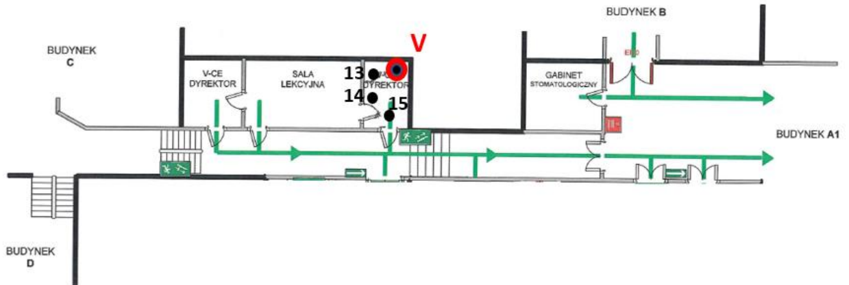
Rys. 1a: Plan rozmieszczenia punktów pomiarowych – parter, budynek A2 A3, kolorem czerwonym oznaczono lokalizację punktów dostępowych
