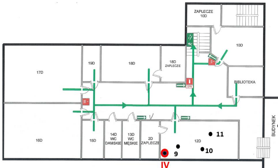
Rys. 1e: Plan rozmieszczenia punktów pomiarowych – piętro 1, budynek D, kolorem czerwonym oznaczono lokalizacje punktów dostępowych
