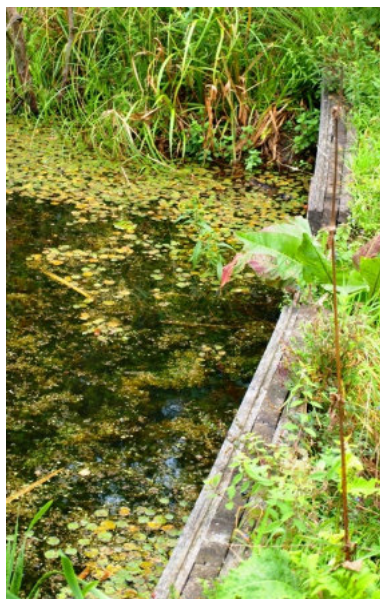
Nawet małe zastawki ulegają naporowi wody jeśli pozbawione są wzmocnień zastrzałem, oczepem i podparciem od dołu umocnieniem. Fot. Z. Filipek Źródło: Archiwum CKPS
