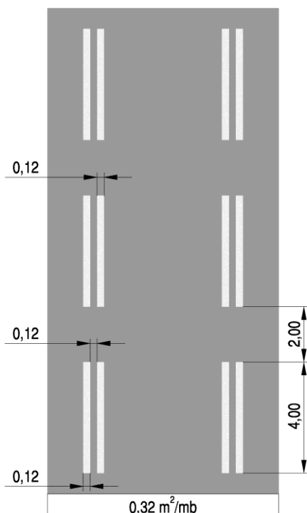
Rys. 2.2.1.11. Znak P-5
