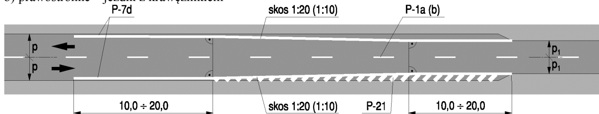
c) dwustronne – jezdni z krawężnikami
