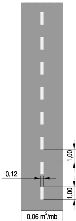
Rys. 2.2.1.4. Znak P-1d
