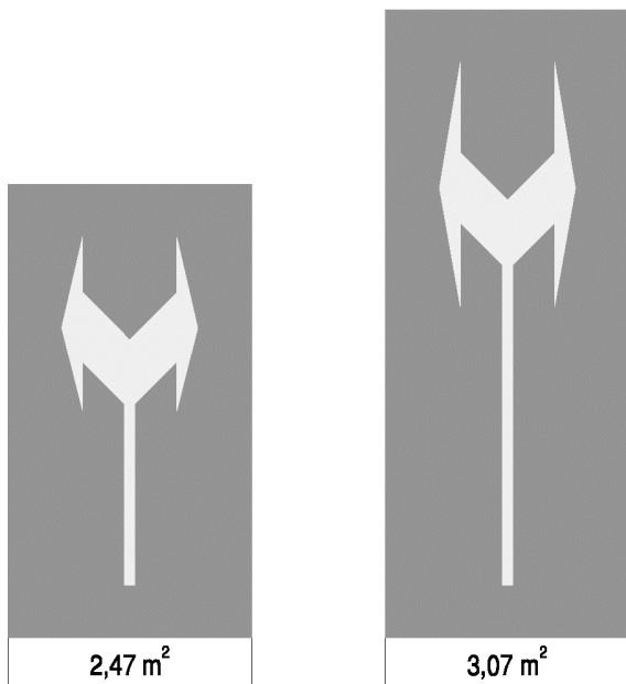
Rys. 3.2.1.8. Znak P-8g:
