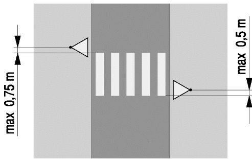
Rys. 7.3.1. Przykłady lokalizacji sygnalizatorów na przejściach dla pieszych:
