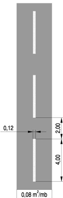
Rys. 2.2.1.12. Znak P-6
