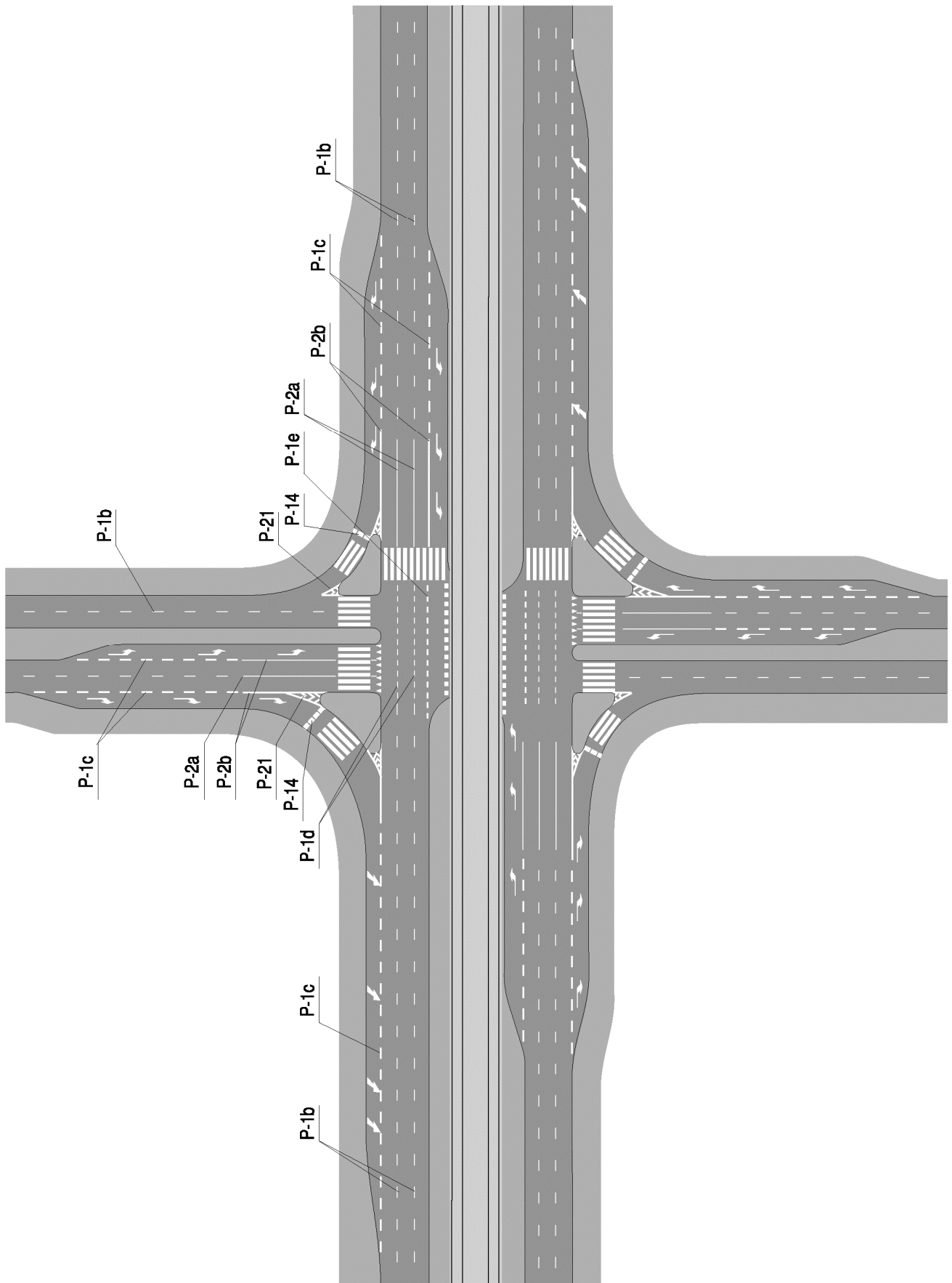
Rys. 8.3.3. Oznakowanie skrzyżowania skanalizowanego
