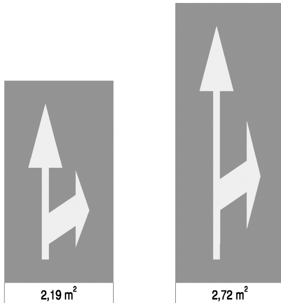
Rys. 3.2.1.7. Znak P-8f:
