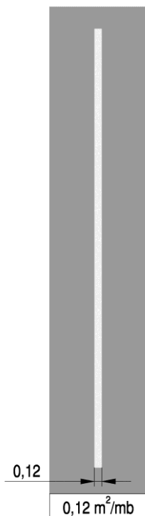
Rys. 2.2.1.6. Znak P-2a
