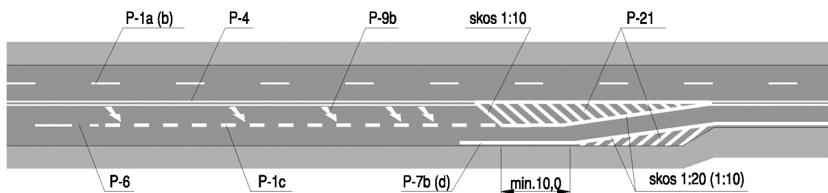
a) na jezdni dwukierunkowej czteropasowej
