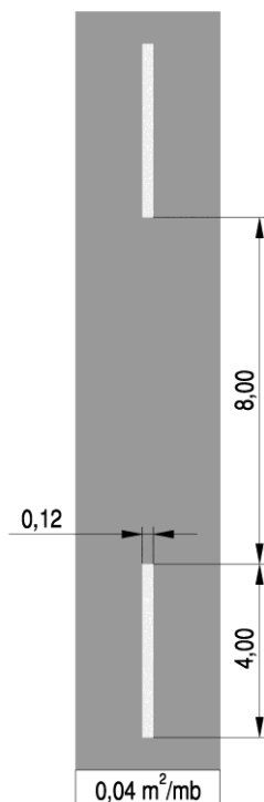
Rys. 2.2.1.1. Znak P-1a
