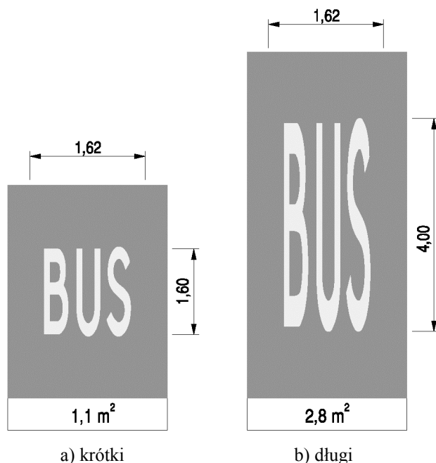
Rys. 5.2.8.1. Znak P-22:
