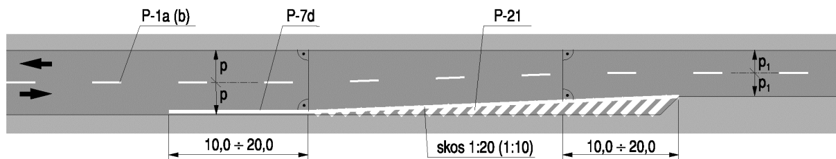
b) prawostronne – jezdni z krawężnikiem
