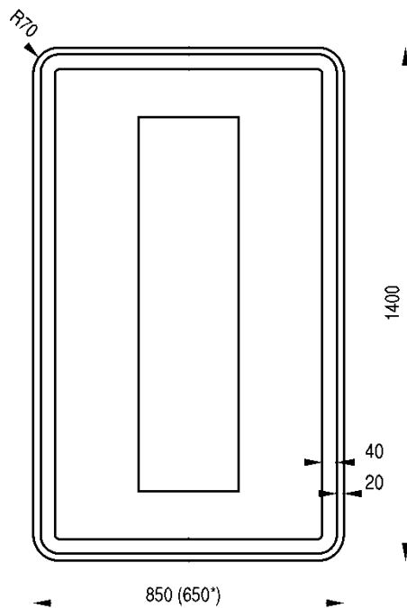
Rys. 10.28. Ekrany kontrastowe prostokątne:
