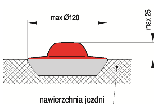
Rys. 6.1.3. Punktowy element odblaskowy o odbłyśniku wielokierunkowym
