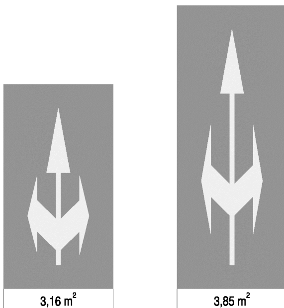
Rys. 3.2.1.9. Znak P-8h:
