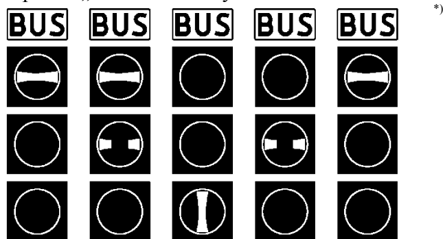
Rys. 4.7.1. Sygnalizator SB z sekwencją sygnałów dla kierujących autobusami
