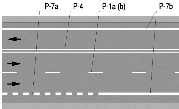
a) z liniami krawędziowymi i poboczem twardym (opaska)
