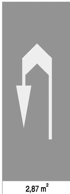
Rys. 3.2.1.4. Znak P-8c
