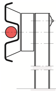
Rys. 2.1.4. Przykład punktowego elementu odblaskowego U-1c umieszczanego na barierze ochronnej
