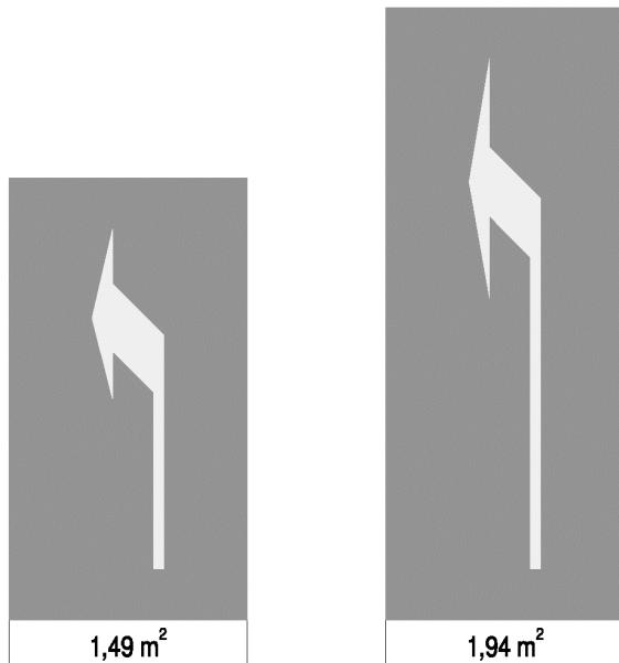
Rys. 3.2.1.3. Znak P-8b:
