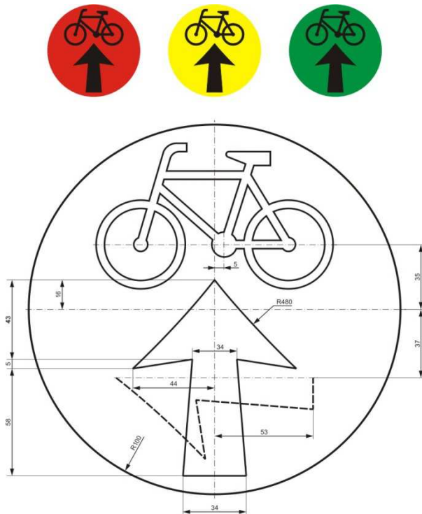
Rys. 10.3. Strzałka kierunku jazdy wprost wraz z symbolem roweru na sygnalizatorze kierunkowym S-3a dla kierujących rowerem; symbol strzałki może wskazywać również kierunki jazdy w prawo oraz w lewo (obróć 90°). Wymiary sylwetki roweru należy zmniejszyć do 75% wymiarów określonych na rysunku 10.1
