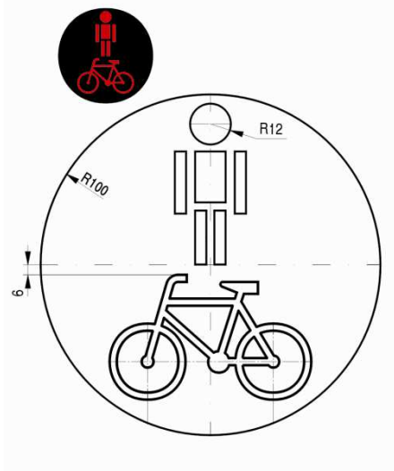
Rys. 10.23. Sylwetki pieszego i rowerzysty wspólnie w sygnale czerwonym; szablon pieszego według konstrukcji na rys. 10.20 należy zmniejszyć o 40%, a szablon roweru według konstrukcji na rys. 10.21 – o 30%
