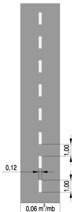
Rys. 2.2.2.3. Znak P-7c
