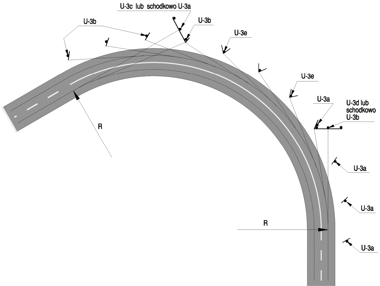
Rys. 2.3.4. Dobór i rozmieszczenie tablic prowadzących U-3 wzdłuż łuku o dużym promieniu i regularnej krzywiznie
