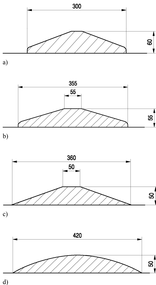
Rys. 8.2.1. Kształt i wymiary w przekroju poprzecznym przykładowych progów podrzutowych:
