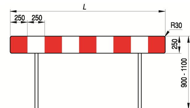
Rys. 11.2.1. Wzory zapór drogowych pojedynczych:
