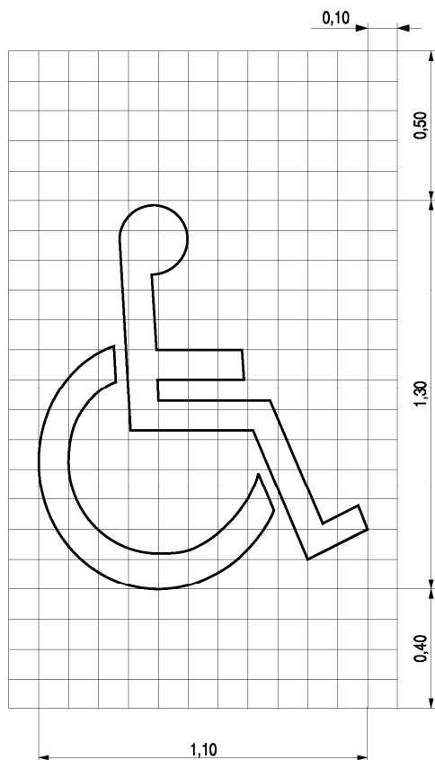
Rys. 5.2.9.2. Znak P-24
