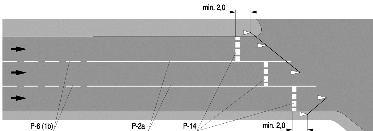
a) bez przejścia dla pieszych
