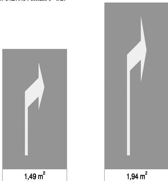
Rys. 3.2.1.5. Znak P-8d:
