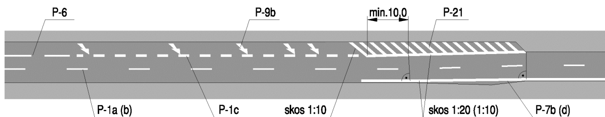
b) na jezdni jednokierunkowej
