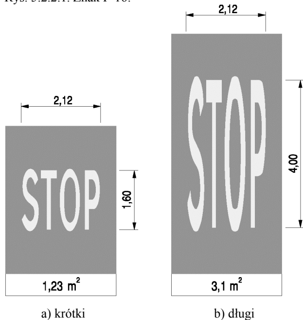
Rys. 5.2.2.1. Znak P-16:
