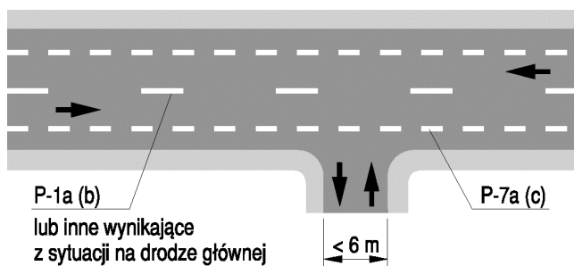
Rys. 7.6.3.1. Kształtowanie linii krawędziowych na zjazdach indywidualnych i publicznych o szer. <math>< 6,0\text{ m}</math>
