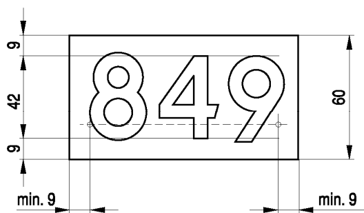
Rys. 2.1.7. Konstrukcja znaku U-1f z numerem drogi
