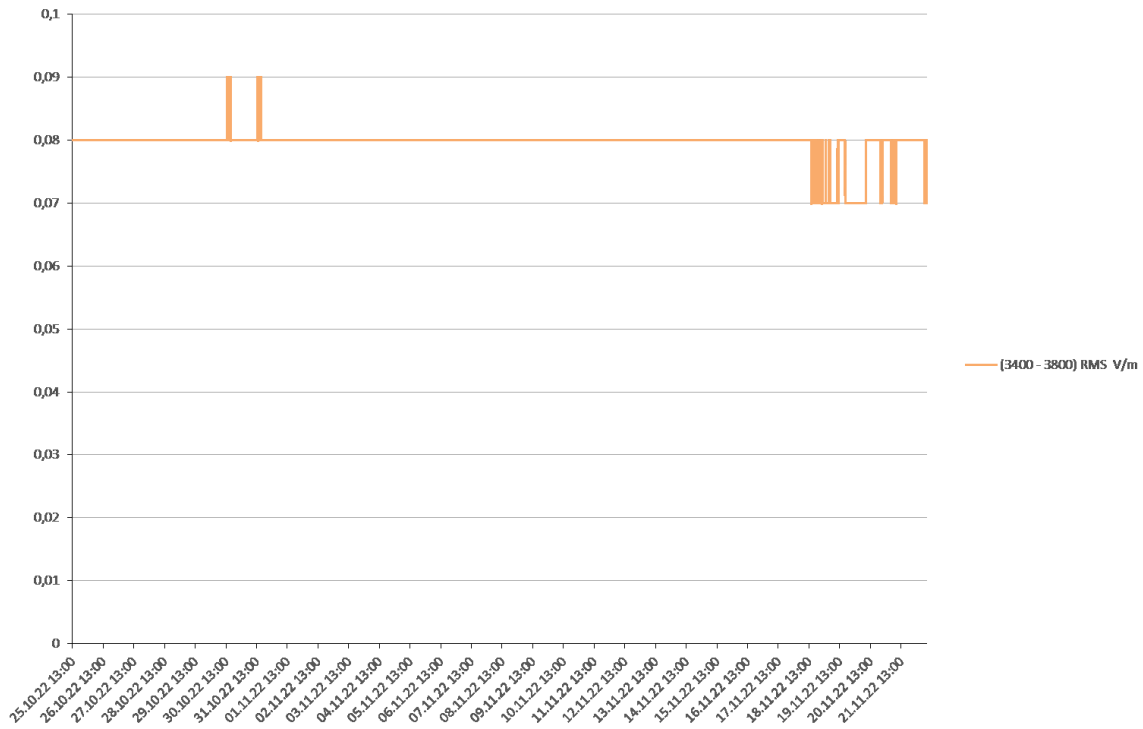
Rys. 23 Wyniki pomiarów: 3400,0 MHz – 3800,0 MHz
