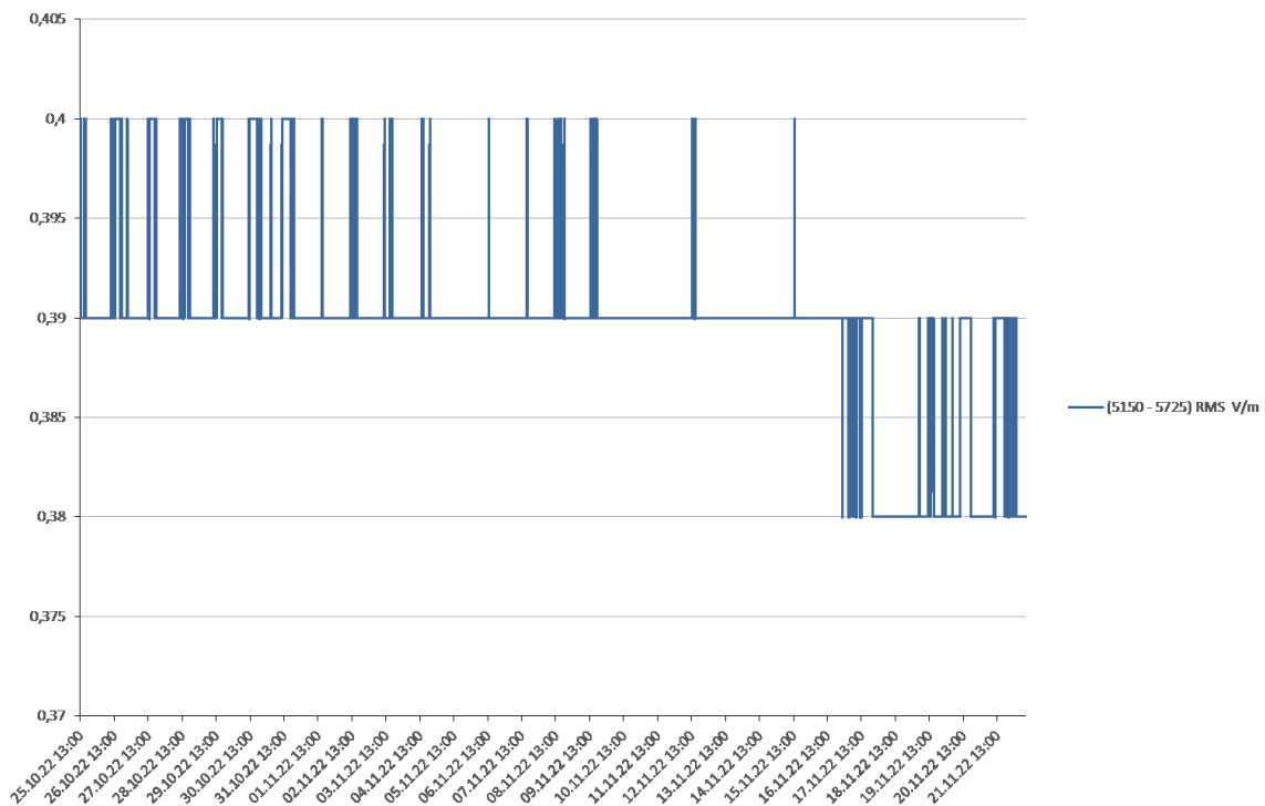
Rys. 24 Wyniki pomiarów: 5150,0 MHz – 5725,0 MHz
