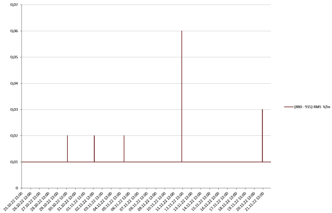
Rys. 13 Wyniki pomiarów: 880,0 MHz – 915,0 MHz
