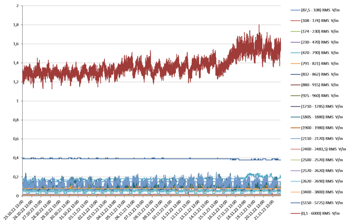
Rys. 4 Wyniki pomiarów dla 20 podzakresów częstotliwości – Wodociągi Jaworzno
