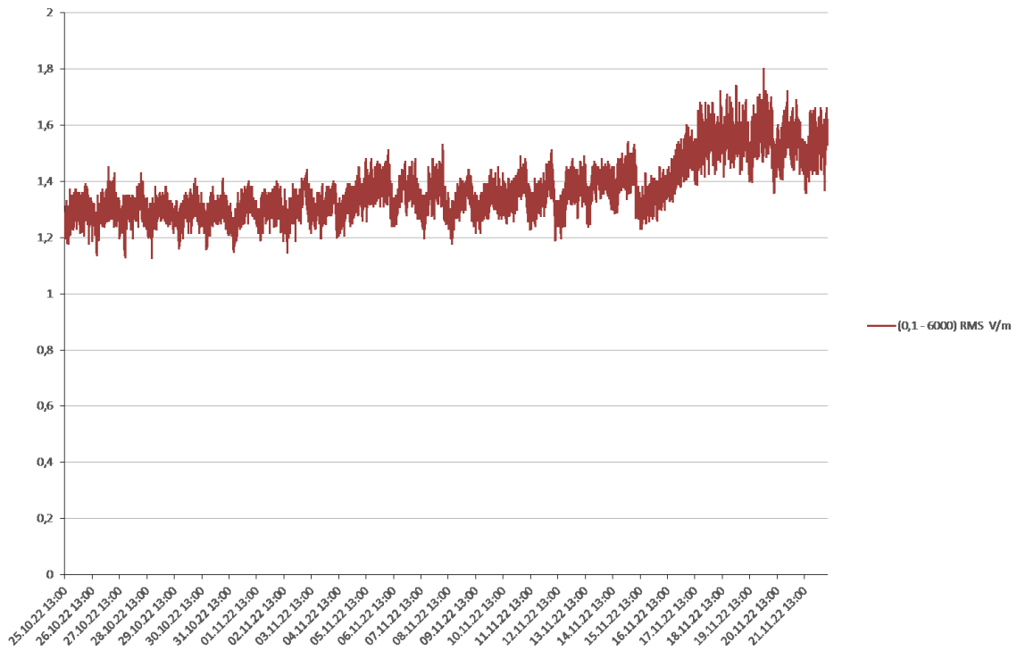
Rys. 5 Wyniki pomiarów: 0,1 MHz – 6000,0 MHz
