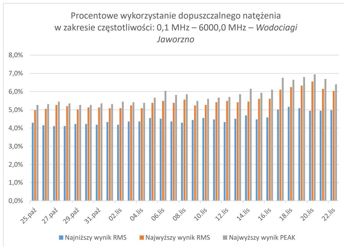
Rys. 25 Procentowe wykorzystanie dopuszczalnego natężenia w zakresie częstotliwości: 0,1 MHz – 6000,0 MHz – Wodociągi Jaworzno
