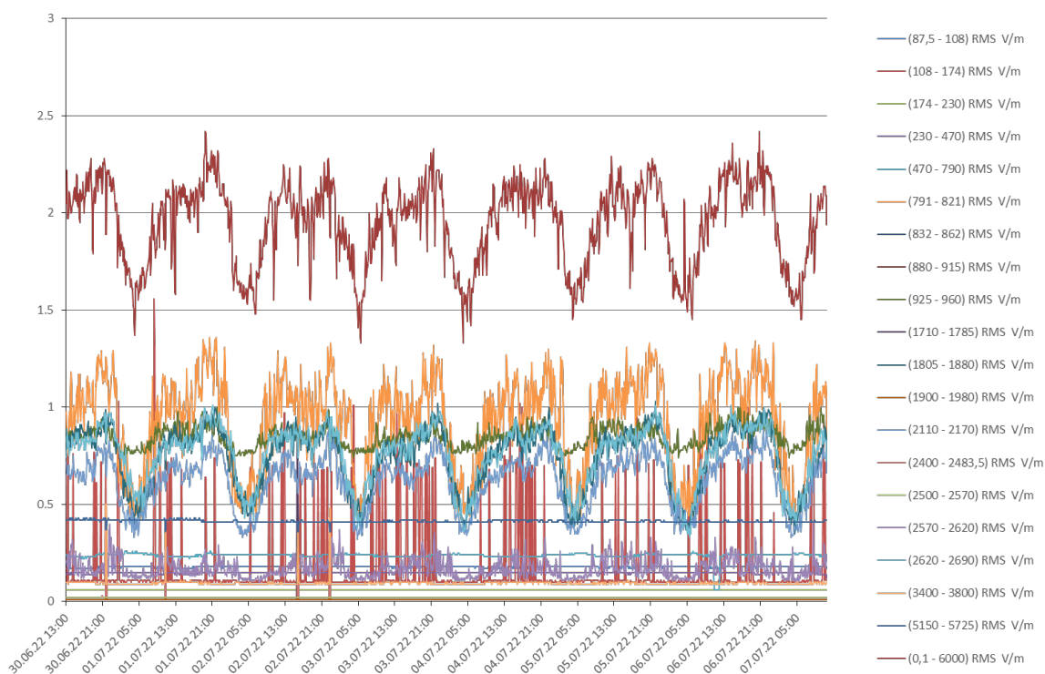
Rys. 8 Wyniki pomiarów dla 20 podzakresów częstotliwości – UM Włocławek
