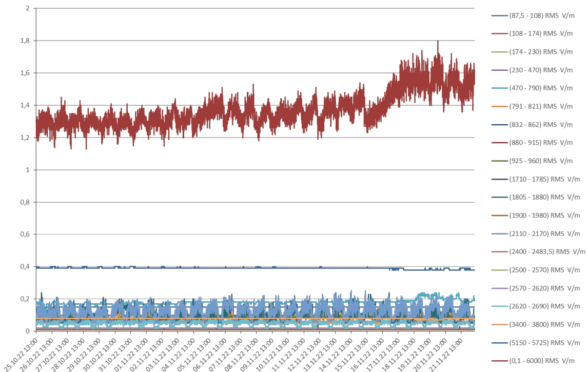
Rys. 11 Wyniki pomiarów dla 20 podzakresów częstotliwości – Wodociąg Jaworzno Najwyższe wartości RMS (wartość średnia) i PEAK (wartość szczytowa), z wyników pomiarów dla wszystkich 20 podzakresów częstotliwości uzyskanych w kolejnych dniach, w poszczególnych lokalizacjach, przedstawiono w Tabl. 4 ÷ Tabl. 7.
