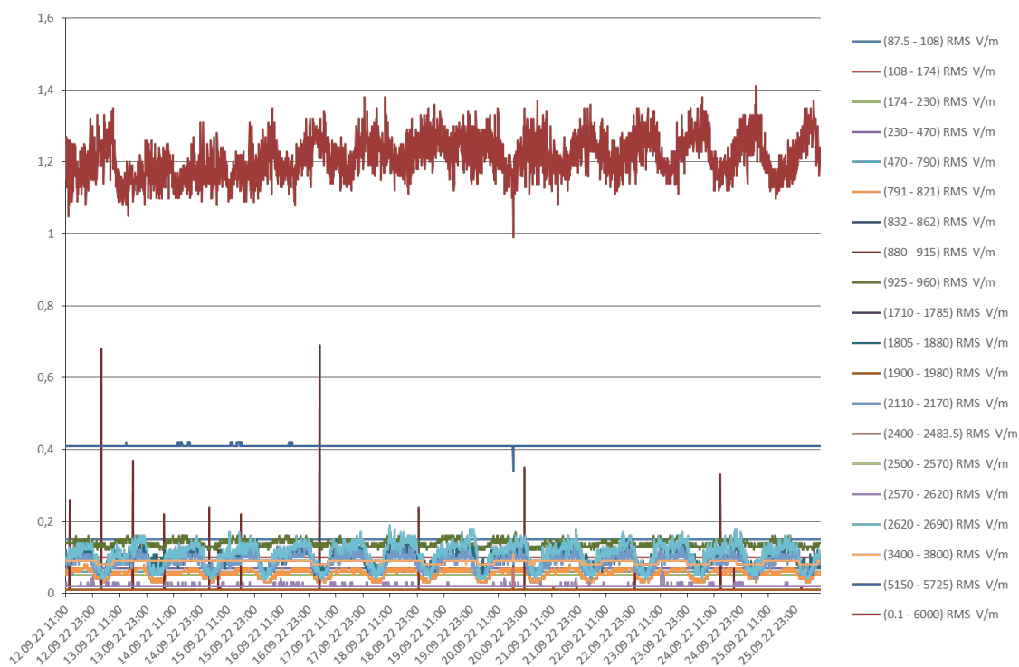
Rys. 9 Wyniki pomiarów dla 20 podzakresów częstotliwości – Szkoła Podstawowa nr 10 w Pruszkowie
