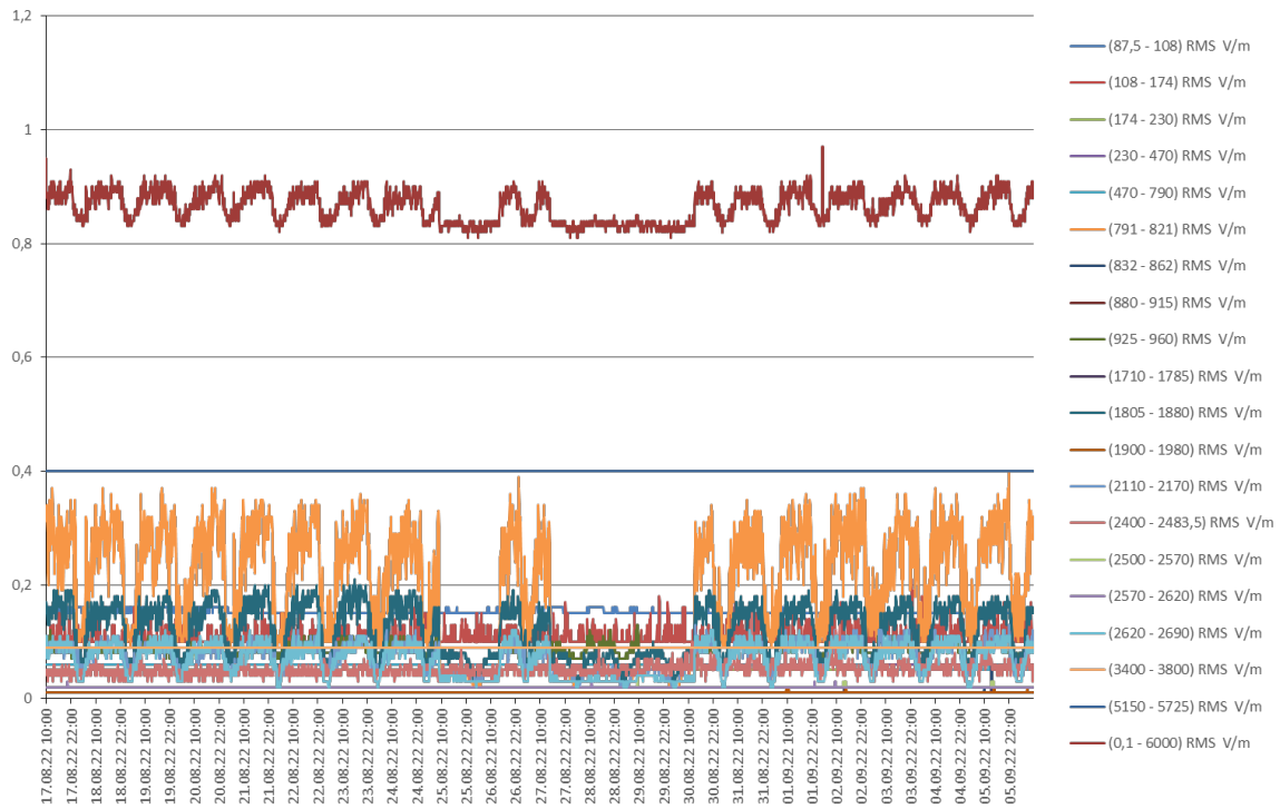
Rys. 10 Wyniki pomiarów dla 20 podzakresów częstotliwości – Szkoła Podstawowa nr 97 we Wrocławiu
