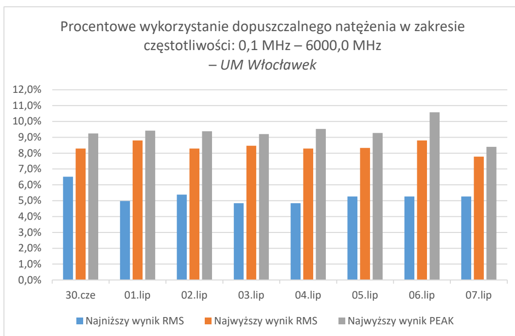
Rys. 12 Procentowe wykorzystanie dopuszczalnego natężenia w zakresie częstotliwości: 0,1 MHz – 6000,0 MHz – UM Włocławek
