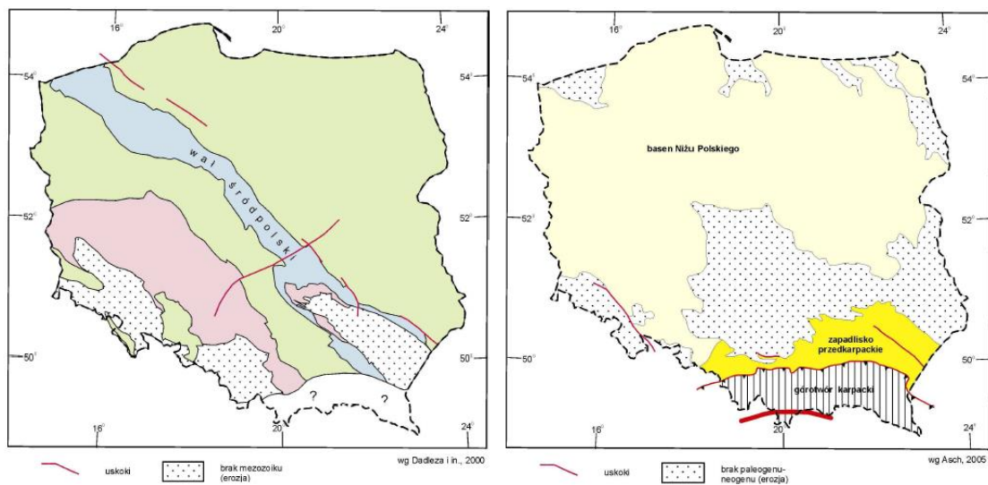
C – mapa bez kenozoiku
