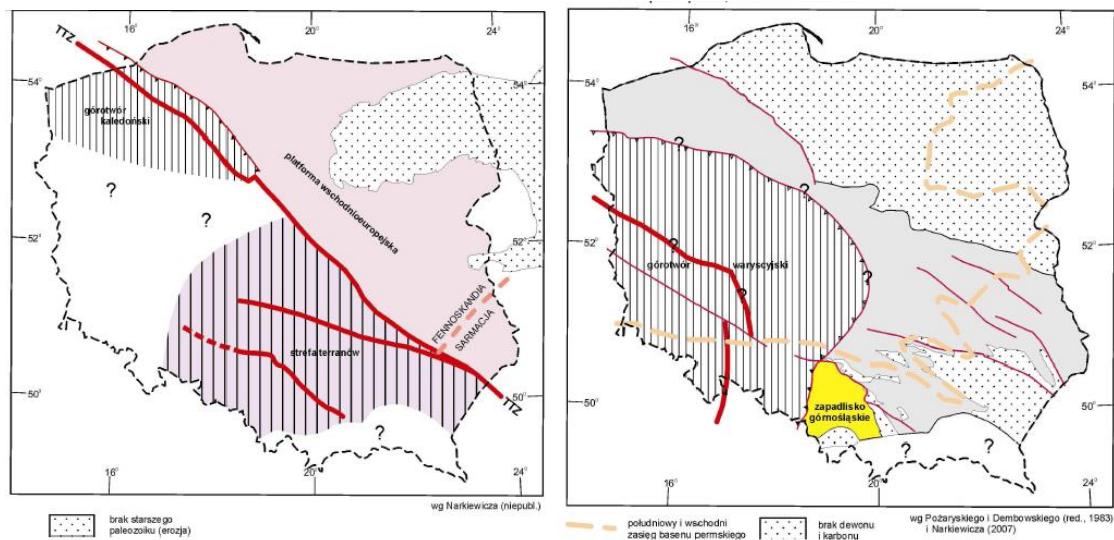
A – mapa poddewońska
