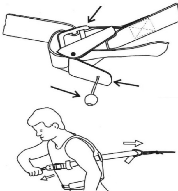
Rys. 1 Budowa i zasada działania bezpiecznej klamry w kamizelce asekuracyjnej
